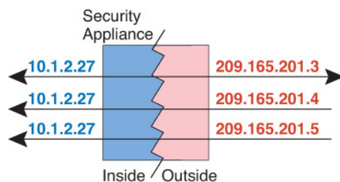
図 7: 一対多のスタティック NAT
