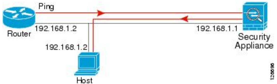
図 3: IP アドレッシングの問題による ping の失敗
