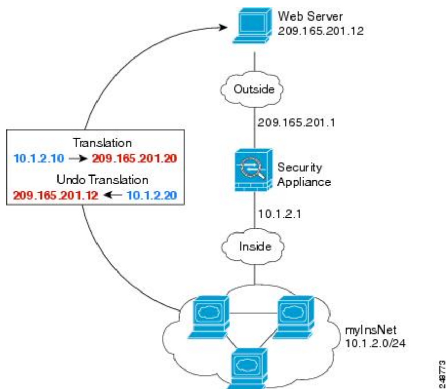
図 2: 内部のダイナミック NAT、外部 Web サーバーのスタティック NAT
