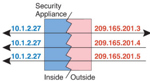
図 7: 一対多のスタティック NAT
