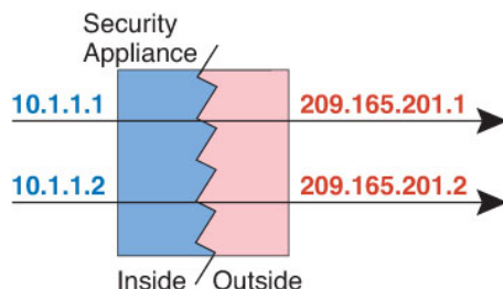
図 2: ダイナミック NAT
