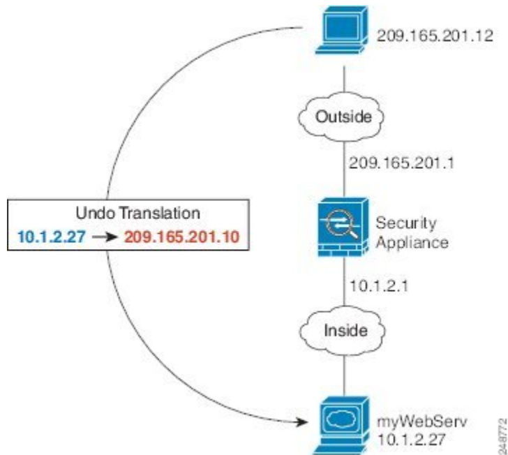
図 1: 内部 Web サーバーの静的 NAT
