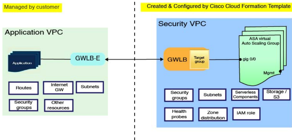
図 2: ASA 仮想 AWS GWLB Auto Scale の導入例の図
