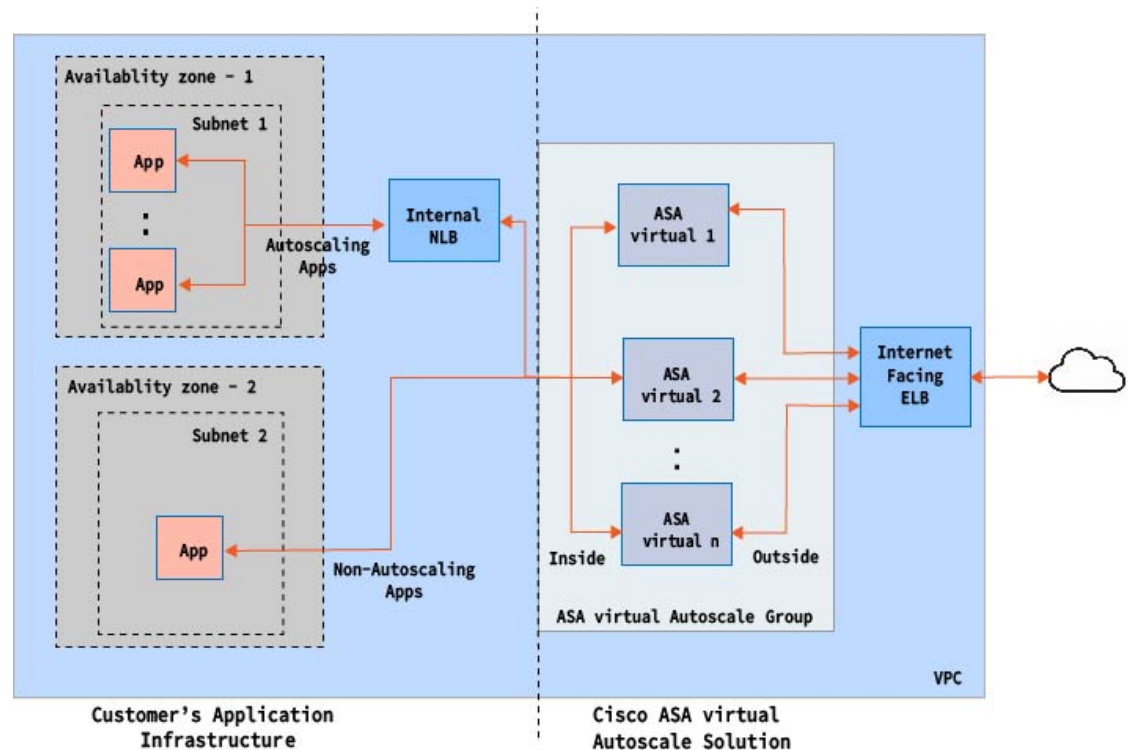
図 1: サンドイッチトポロジを使用した ASA 仮想 Auto Scale の導入例の図
