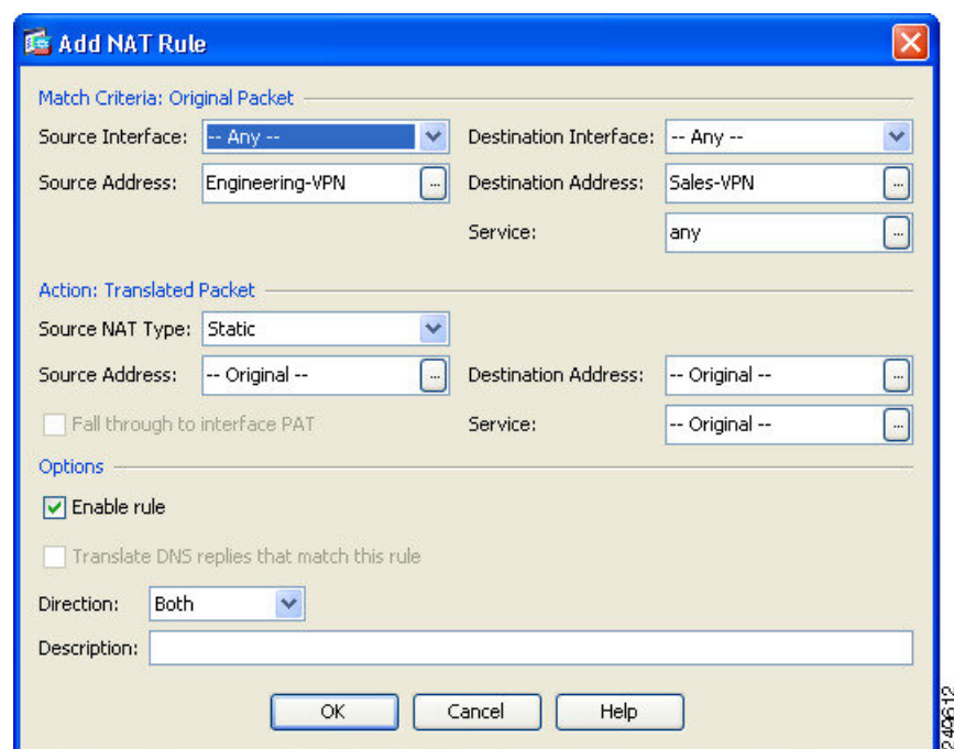
図 1: [Add NAT Rule] ダイアログ ボックス
