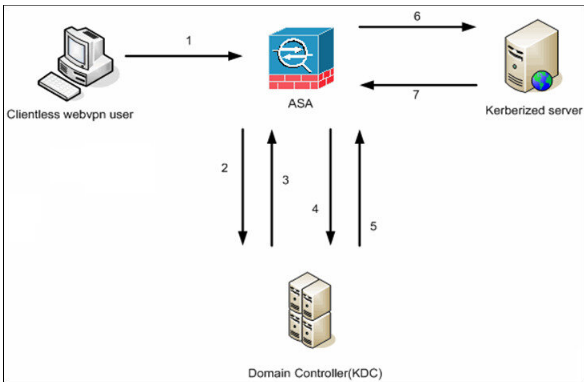
図 10: KCD プロセス
