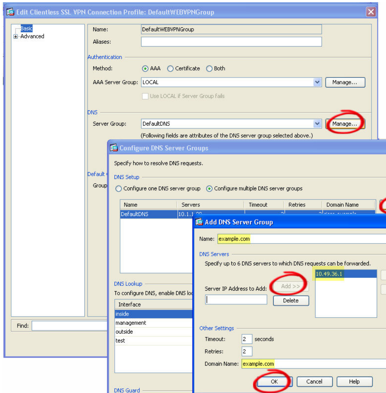
図 9: ポート転送の DNS サーバー値の例
