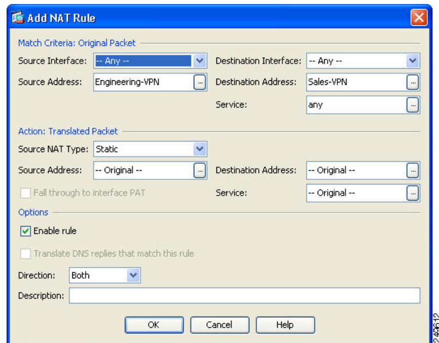
図 2: [Add NAT Rule] ダイアログ ボックス
