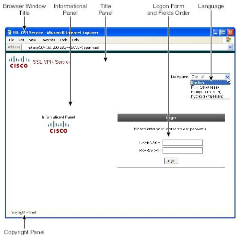
図 11: クライアントレス ログイン ページのコンポーネント
