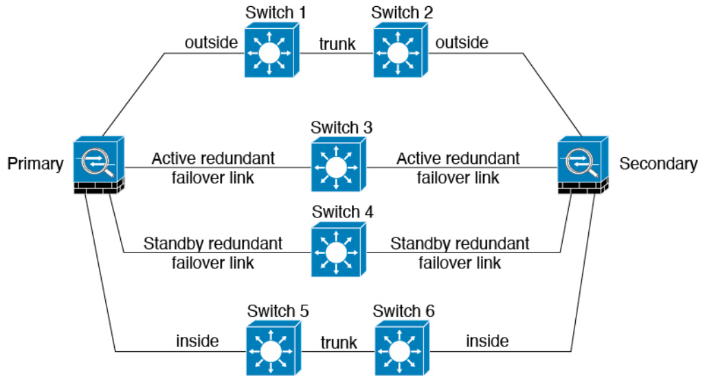
図 7: Inter-Switch Link (ISL) を使用した接続
