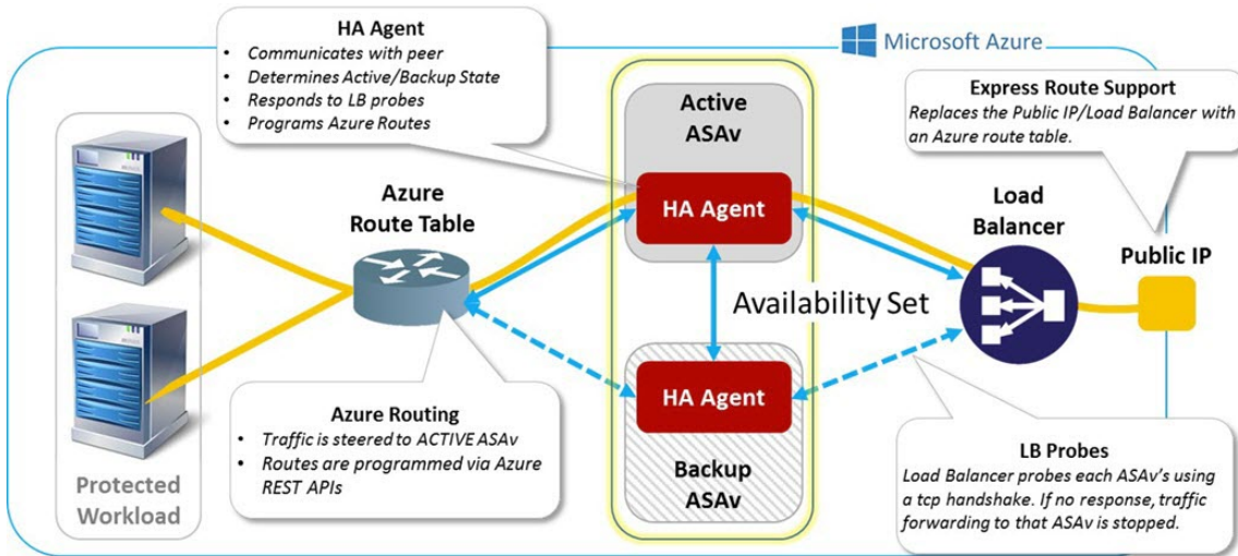
図 1: Azure での ASAv HA 展開
