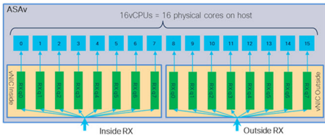
図 5: 16 コア ASA RSS RX キュー
