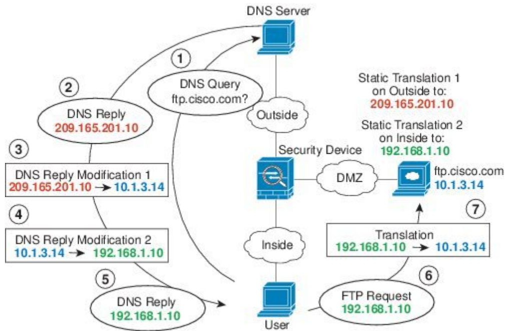
図 17: DNS 応答修正：別々のネットワーク上の DNS サーバ、ホスト、およびサーバ
