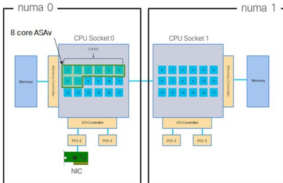
図 5: 8 コア ASAv NUMA アーキテクチャの例
