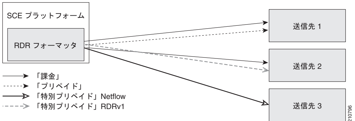
図 8-6 送信先の設定 : 3 つのカテゴリおよび 2 つのプロトコル
