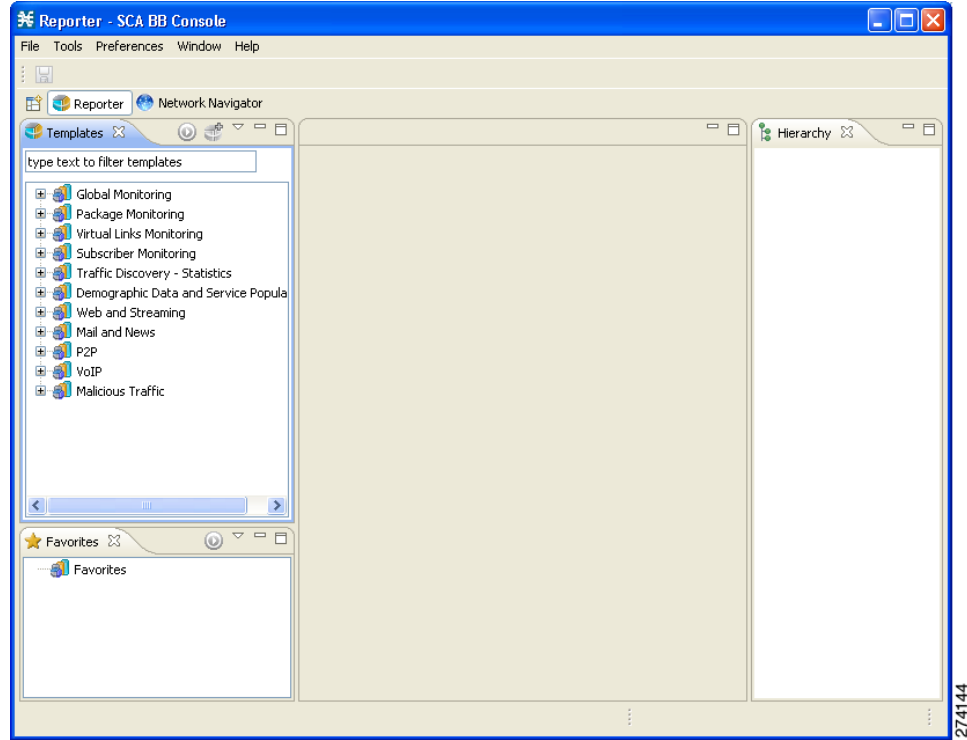
図 C-2 Reporter ツール
