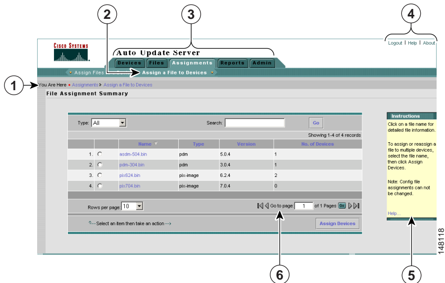
図 1-1 AUS GUI
