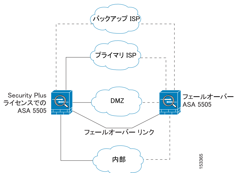
図 5-2 Security Plus ライセンスでの ASA 5505 適応型セキュリティ アプライアンス
