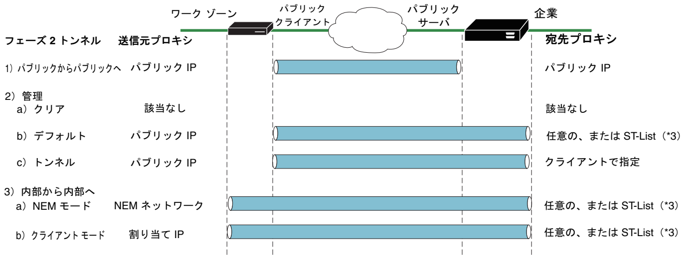
図 8-1 Cisco ASA 5505 用の Easy VPN ハードウェア クライアント トンネリング オプション
