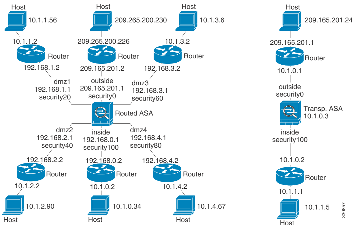
図 14-1 インターフェイス、ルータ、およびホストを含むネットワーク図
