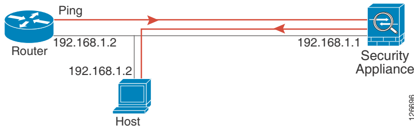
図 14-3 IP アドレッシングの問題による ping の失敗
