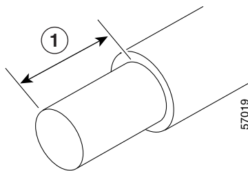
図 17 Cisco ASR 1002-X ルータの +24 V DC 電源モジュールの導線と絶縁体
