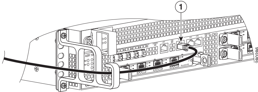
図 8 Cisco ASR 1002-X 統合ルータ プロセッサのイーサネット管理ポート コネクタ
