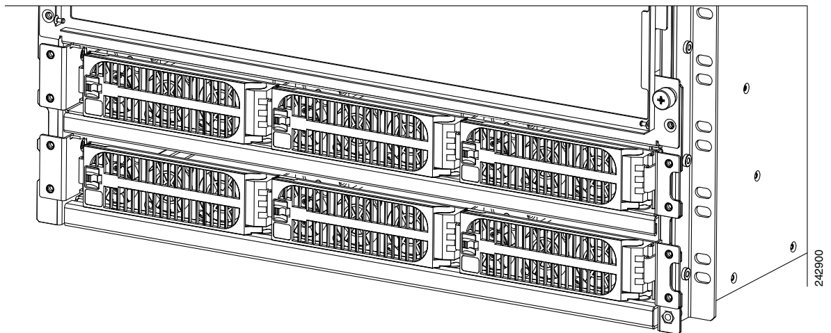
図 1-13 電源シェルフのシステム正面図
