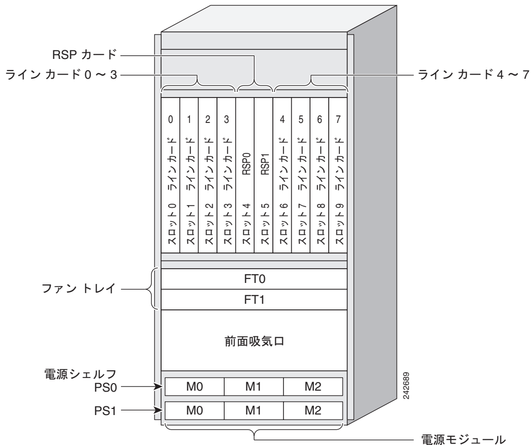
図 1-10 ASR 9010 ルータ スロット ID 付番
