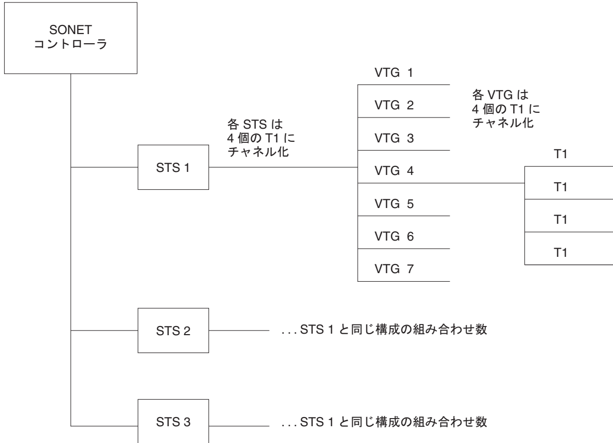
図 12 SDH AU3 パス
