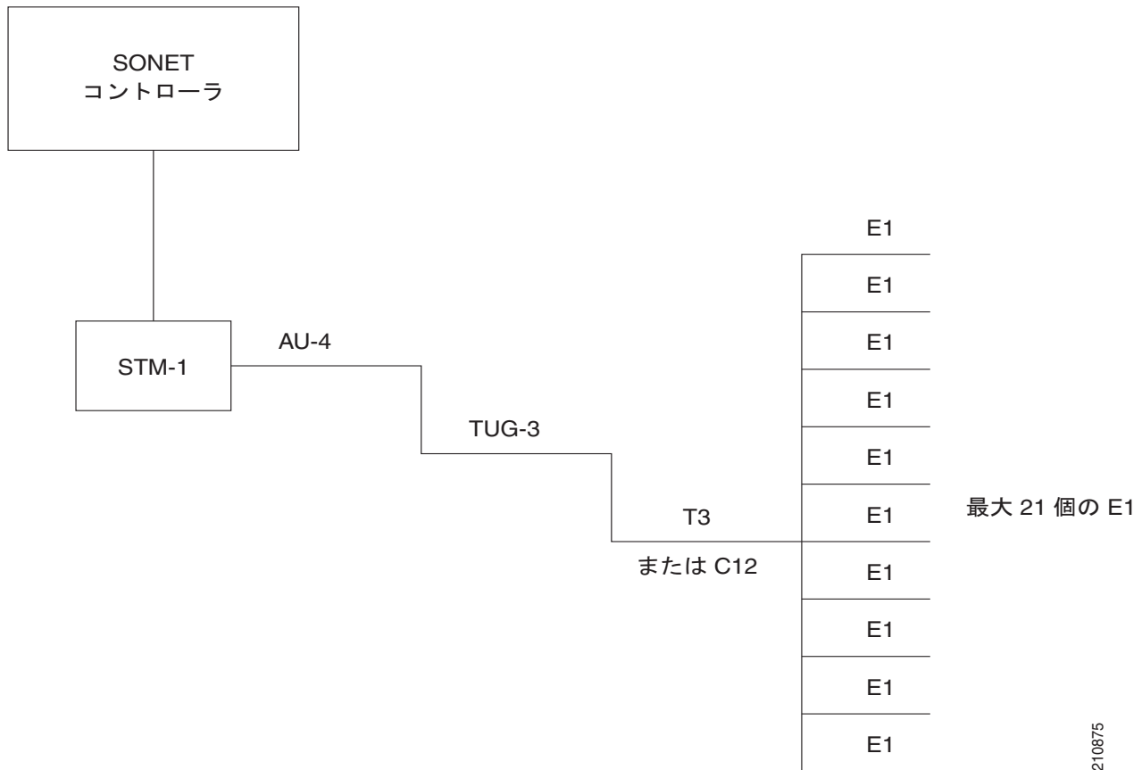
図 13 SDH AU4 パス
