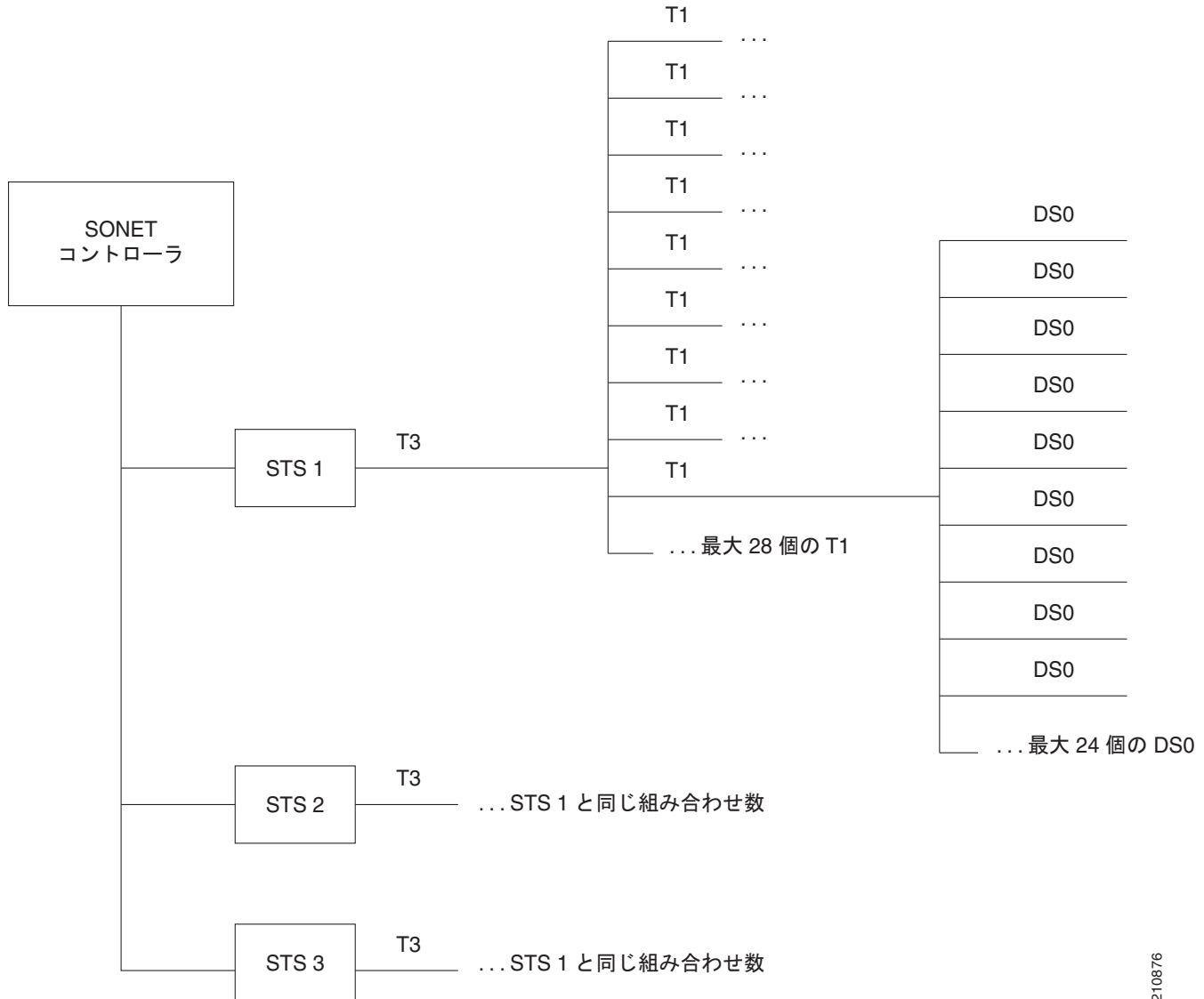
図 11 SONET VTG チャネライズド パス
