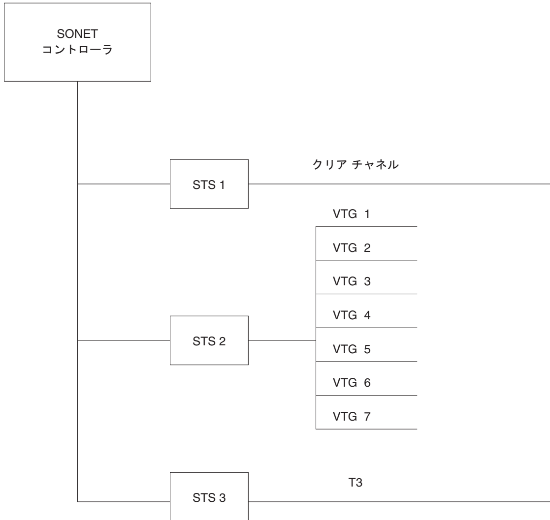
図 10 SONET T3 チャネライズド パス
