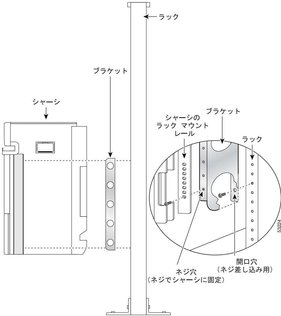
図5 センターマウント ラックマウント ブラケット
