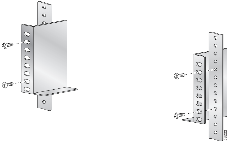
図 4 ラックマウント ブラケット
