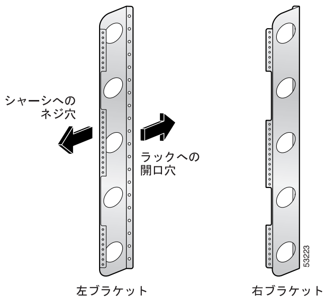
図 2 センターマウント ブラケット
