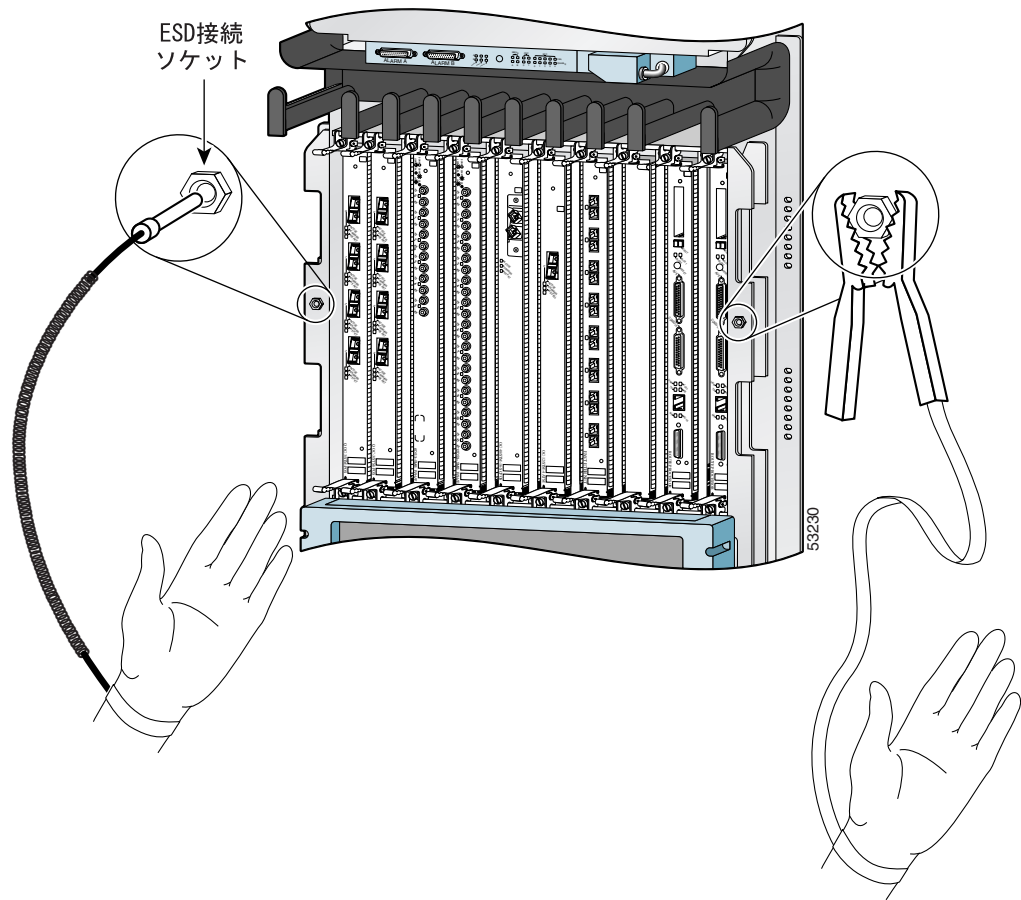
図3 静電気防止用リストストラップのシャーシへの接続
