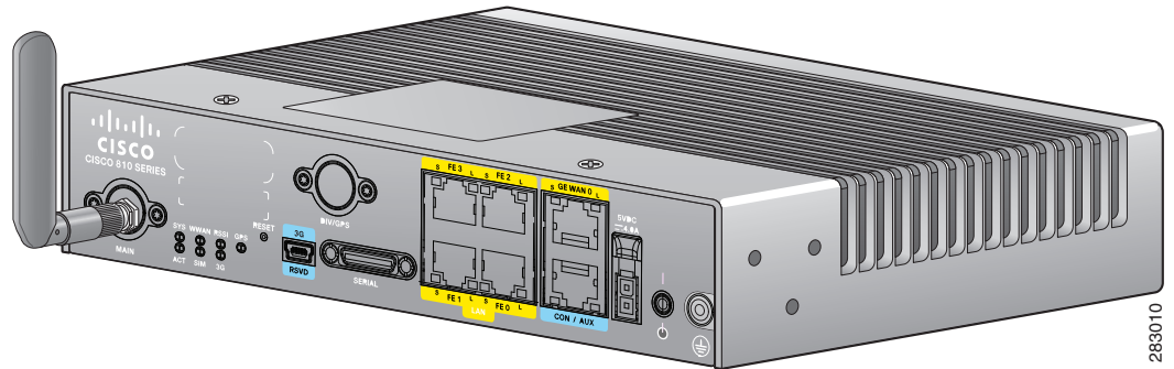
図 1-1 Cisco 819HG サービス統合型ルータ
