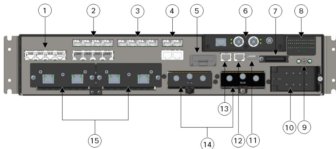
図 2: IR8340 ルータの前面パネル
