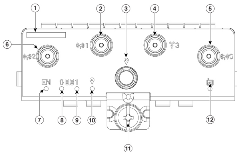
図 8: 5G プラガブルインターフェイス モジュール - P-5GS6-GL
