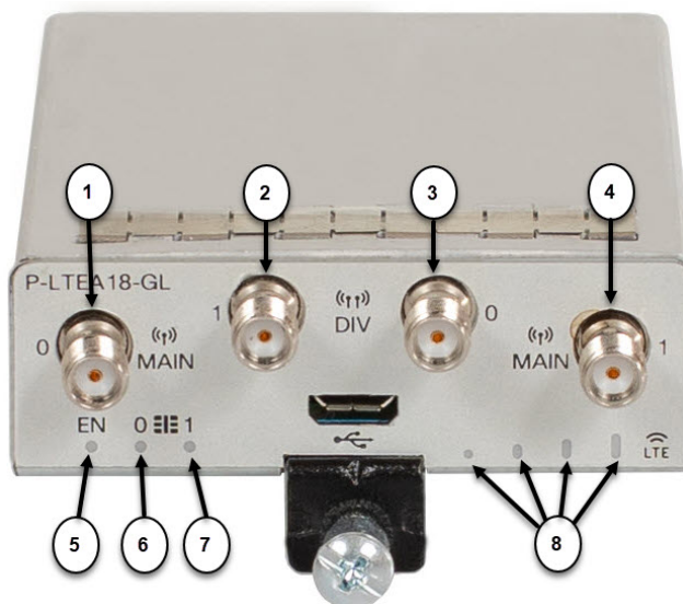
図 7: LTE プラガブル P-LTEAP18-GL
