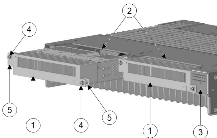
図 10: IR8340 ルータ (両方の電源モジュールを装着)
