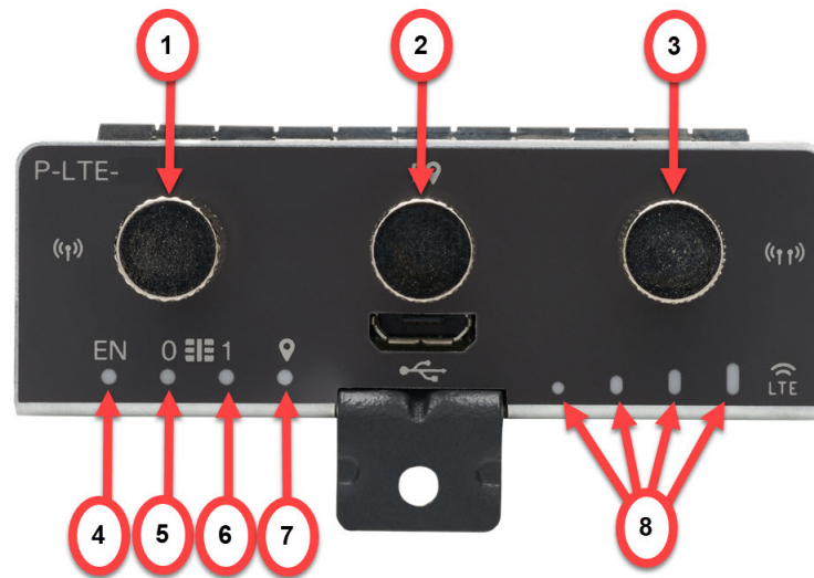
図 5: PIM モジュール
