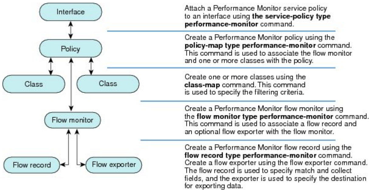
図 11 : Cisco Performance Monitor のコンポーネント
