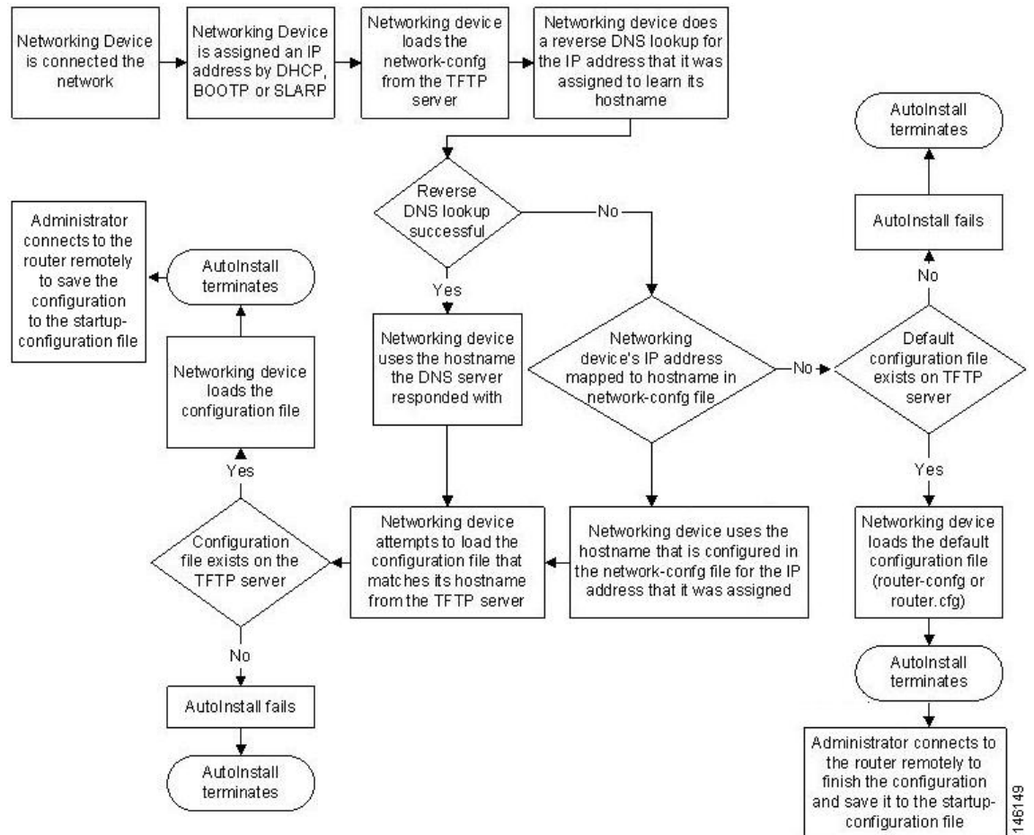
図 7: 自動インストール プロセスのフローチャート (コンフィギュレーション ファイル使用)
