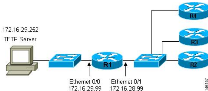
図 8: 特定のデバイスに対する自動インストールコンフィギュレーション ファイルを割り当てるためのネットワーク トポロジ
