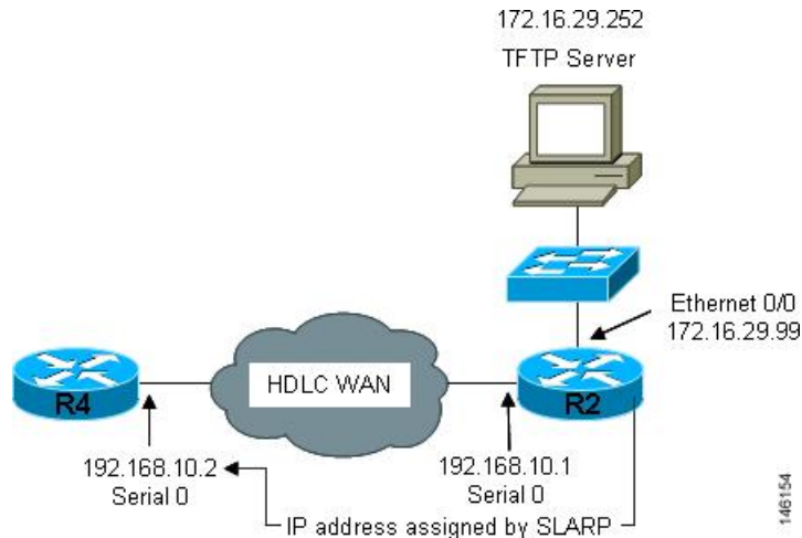
図 2: SLARP を使用した新しいデバイスへの IP アドレスの割り当て
