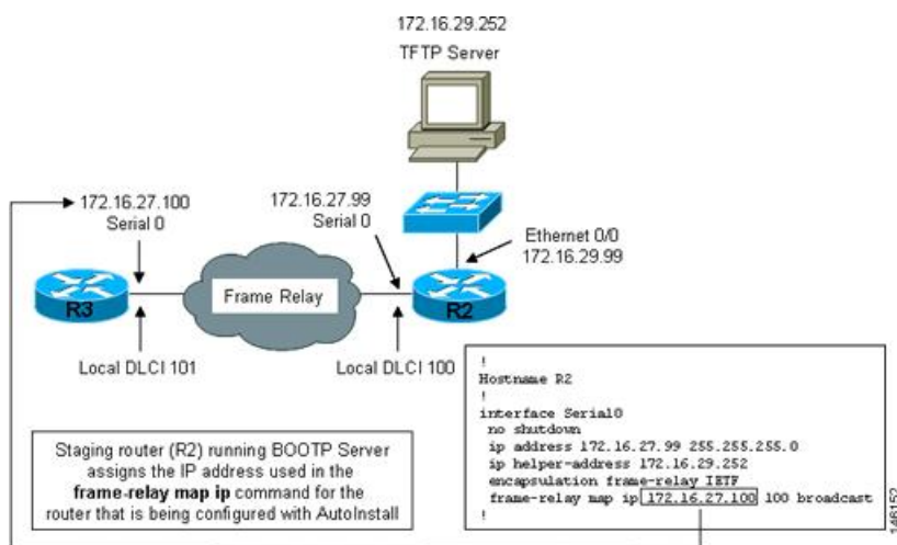
図 3: フレーム リレー ネットワークを介した自動インストールで BOOTP を使用する例
