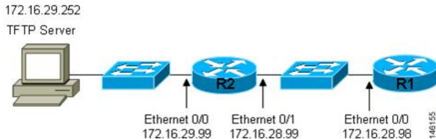
図 4: ステージングルータが必要な自動インストールの例
