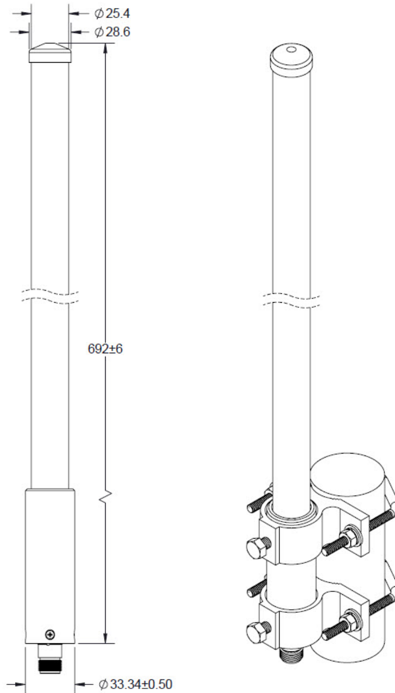
図 2: 寸法
