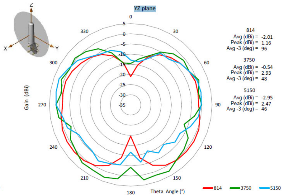
YZ 平面
