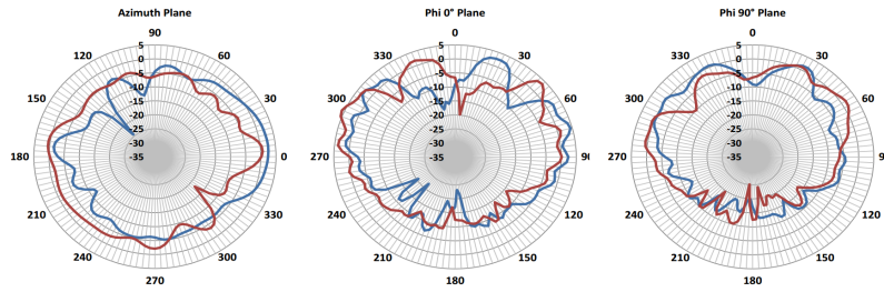
図 14: 5275 MHz WLAN アンテナ放射パターン
