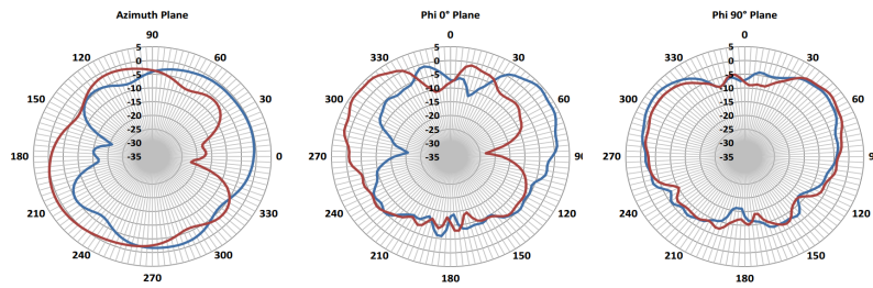
図 11: 2500 MHz WLAN アンテナ放射パターン
