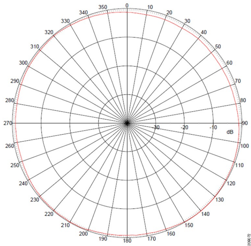
図 3: 方位角面内放射パターン (5 GHz)
