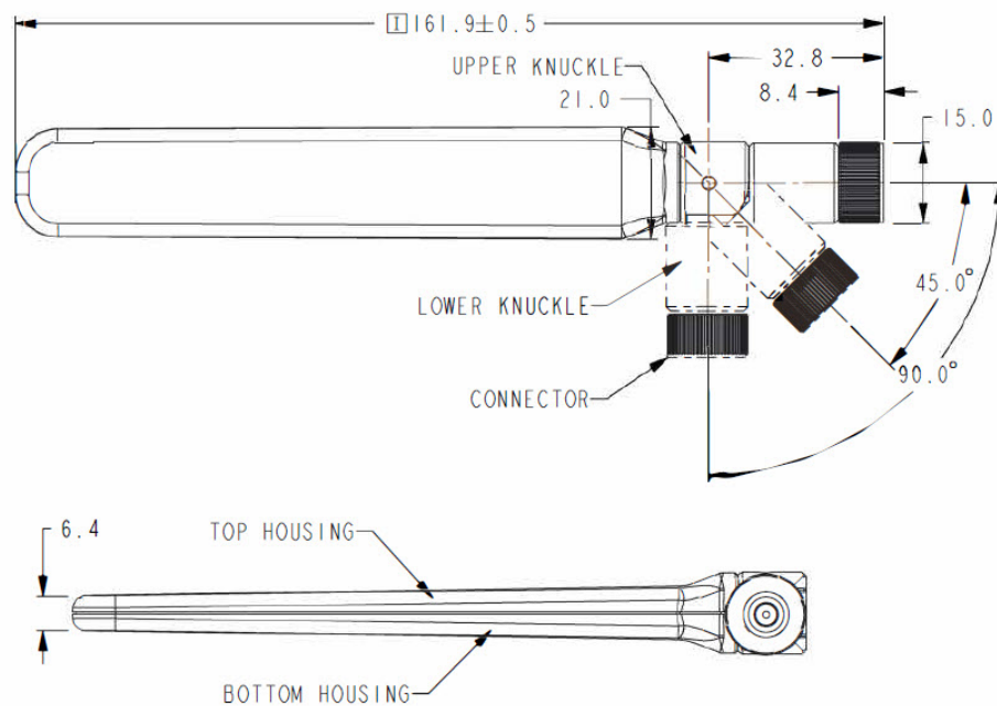
図 2: 機械図面
