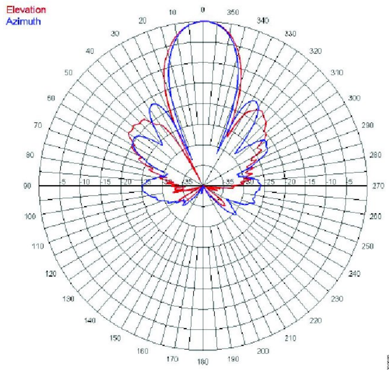
図 2: フラットパネル WiMAX アンテナ放射パターン - ローバンド
