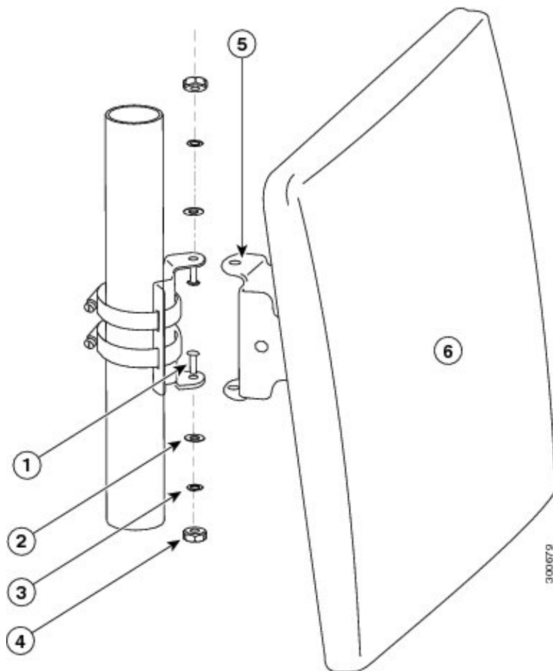
図 4: アンテナの取り付け
