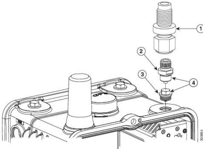
図 5: ケーブルの接続
