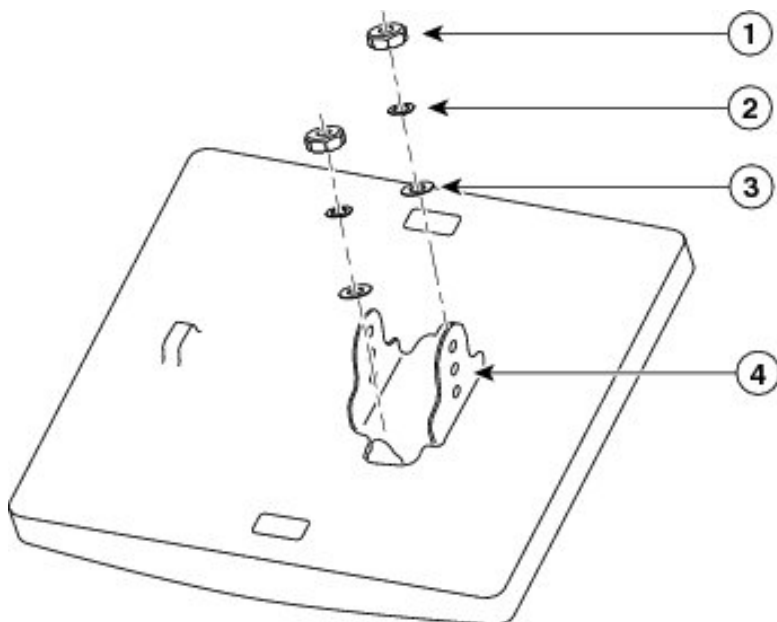
図 3: アンテナ詳細
