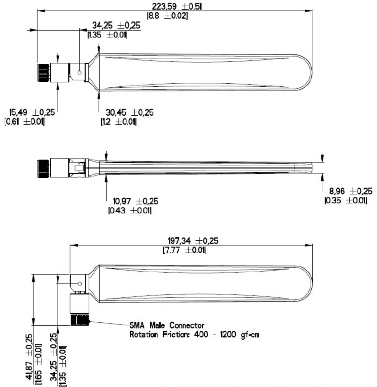
図 2: 機械図面
