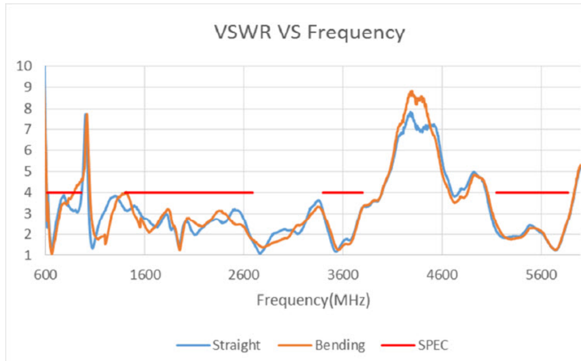
図 3: VSWR と周波数
