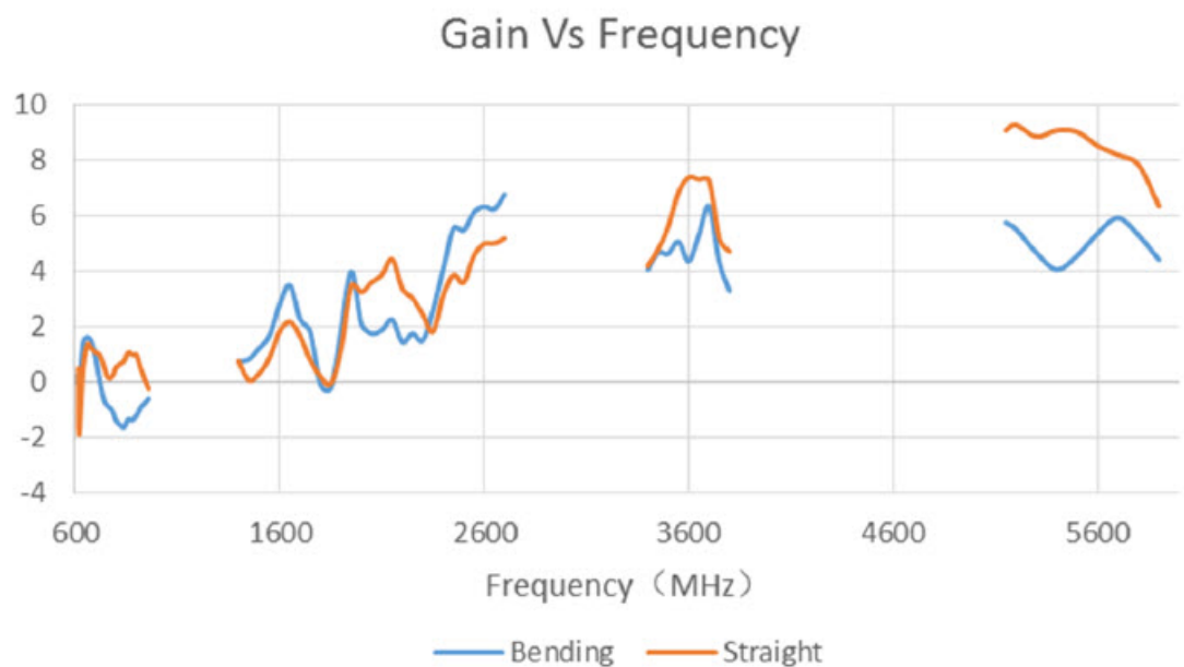
図 5: 利得と周波数
