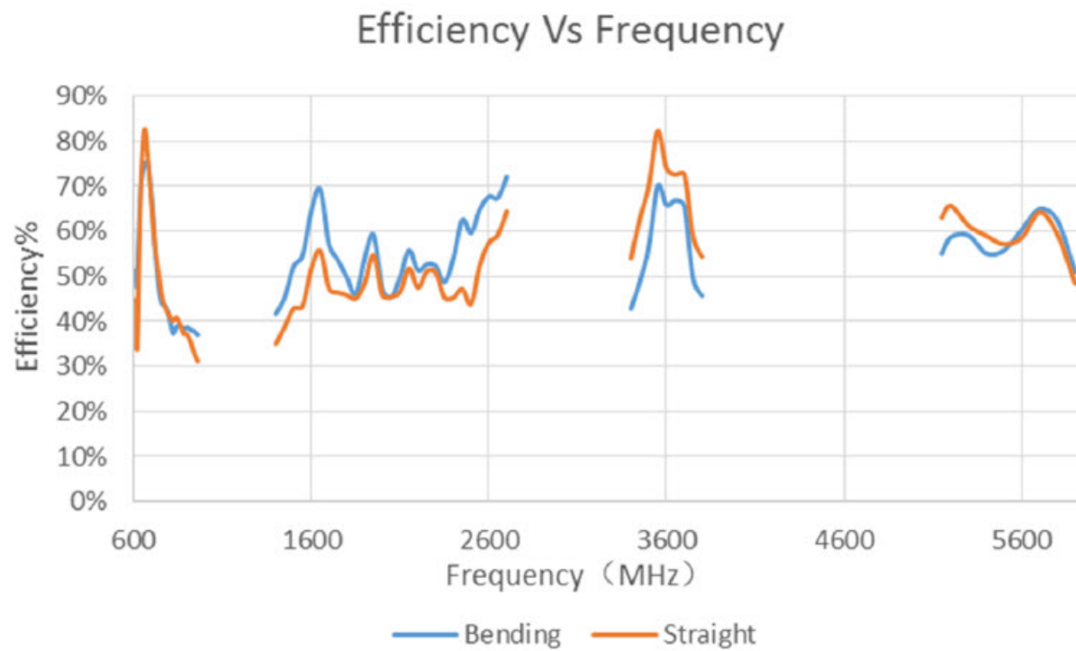
図 6: 効率と周波数
