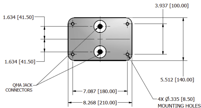
図 3: 底面図
