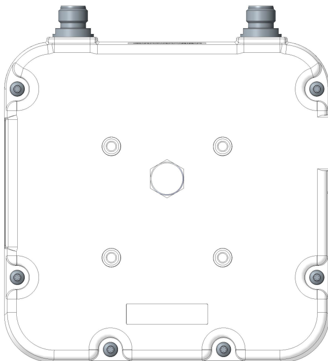
図 4: アンテナ底面
