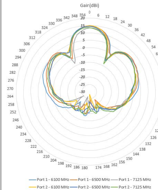
図 7: 6 GHz 放射パターン - 水平面 (X-Z)
