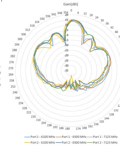
図 8: 6 GHz 放射パターン - 垂直面 (Y-Z)
