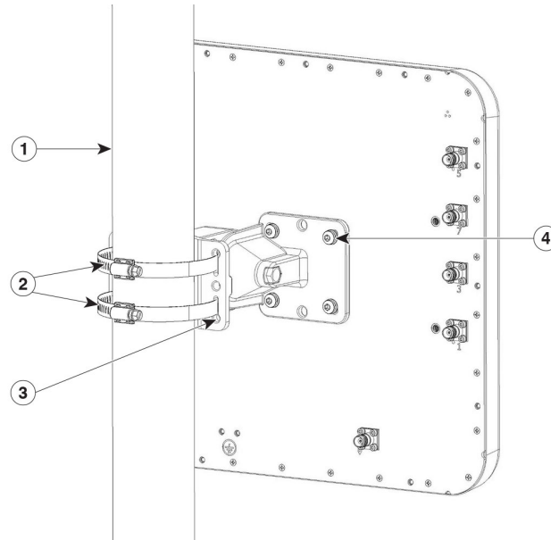
図 18: ピボット付き取り付けブラケットを使用して支柱に取り付けられたアンテナ
