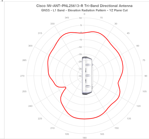
図 13: GNSS 仰角、YZ 平面
