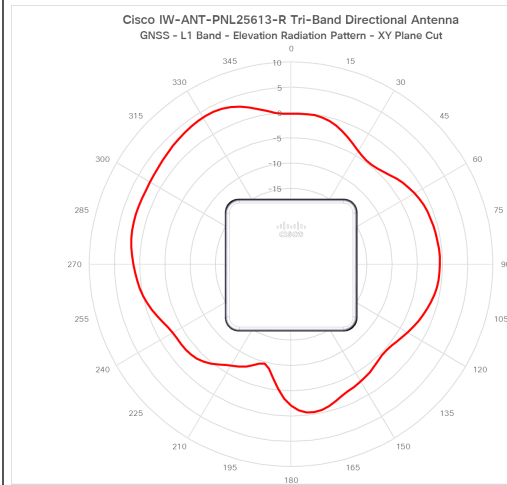
図 12: GNSS 仰角、XY 平面
