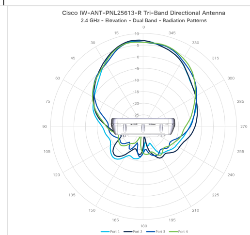
図 7: 2.4 GHz 仰角
