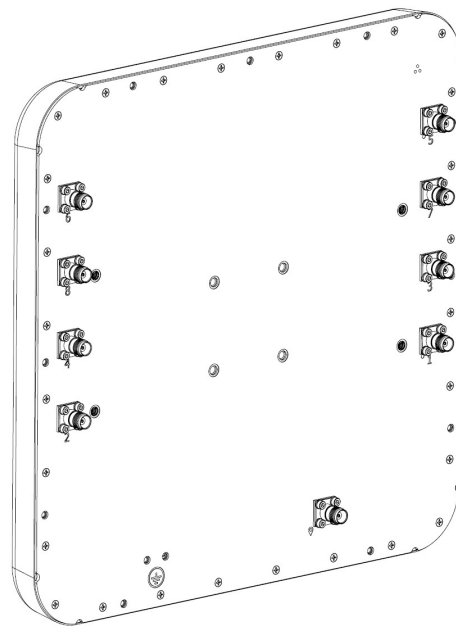
図 2: アンテナ背面図
