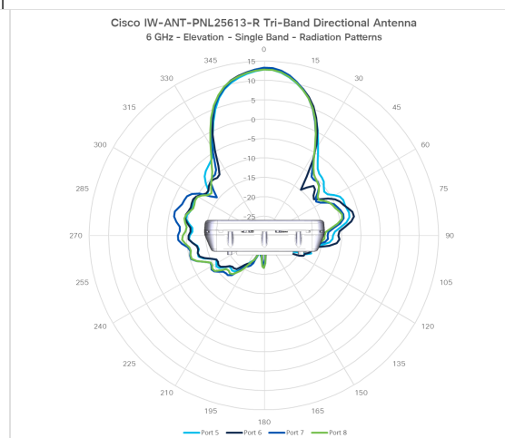
図 11: 6 GHz 仰角
