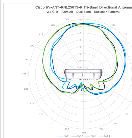
図 6: 2.4 GHz 方位角
