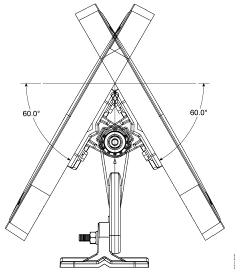
図 22: 仰角調整
