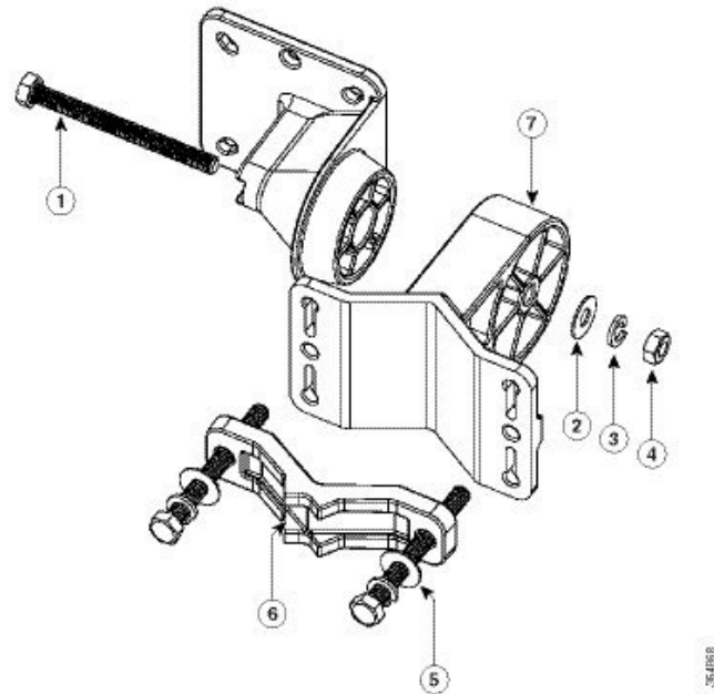
図 15: ピボット取り付けの組み立て図
