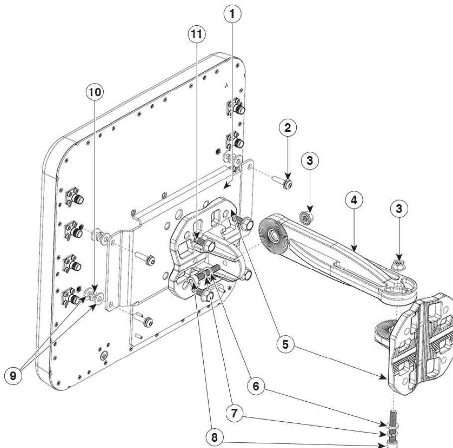
図 23: アンテナおよびブラケット金具のアセンブリの分解図
