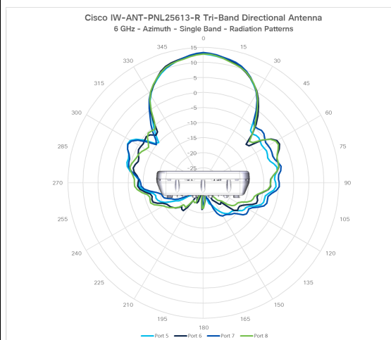
図 10: 6 GHz 方位角
