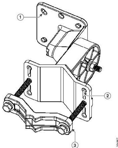
図 19: 支柱取り付けクランプ付きのピボット付き取り付けキット
