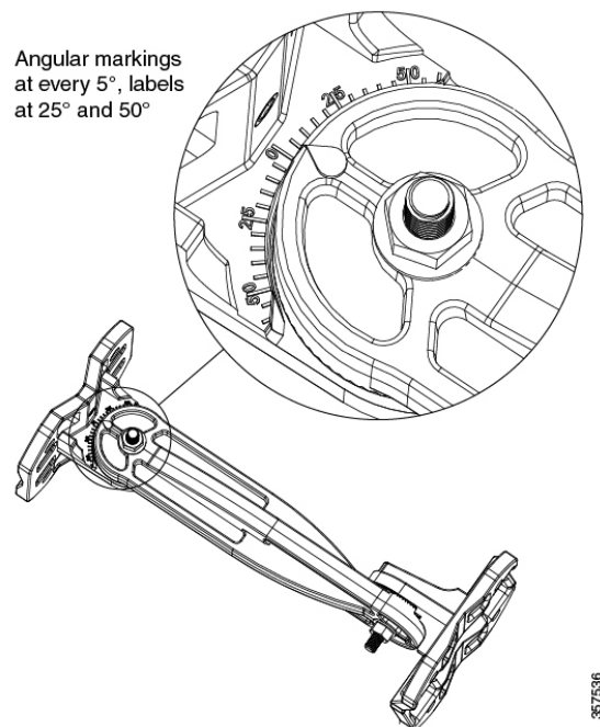
図 20: 方位角調整ピボットおよび仰角調整ピボットの拡大図
