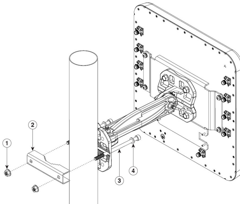
図 24: 支柱取り付け用のアンテナ ブラケット ホース留め金アセンブリ
