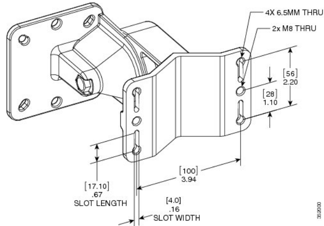
図 15: ピボット取り付けの組み立て図
