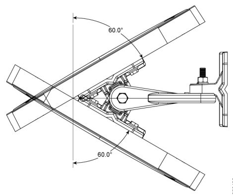
図 22: 仰角調整
