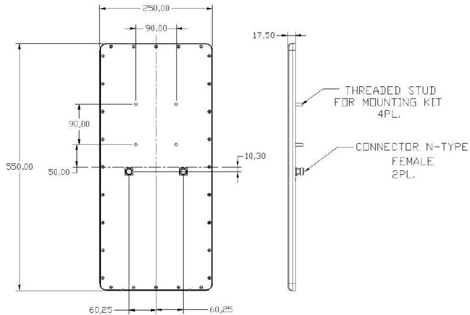
図 2: 機械図面
