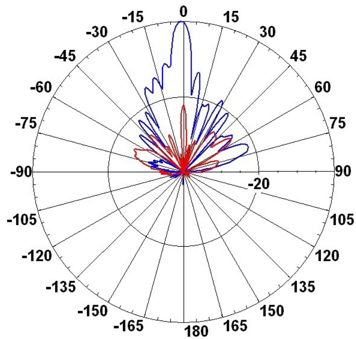
図 4: 仰角面内放射パターン中帯域周波数5.25 GHz
