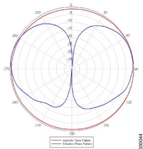
図 1: 2.4 GHz の方位角面および仰角面パターン
