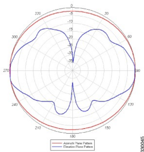
図 2: 5 GHz の方位角面および仰角面パターン
