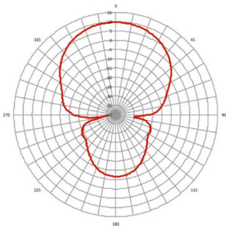
図 7: 910 MHz アンテナ放射パターン - 垂直面
