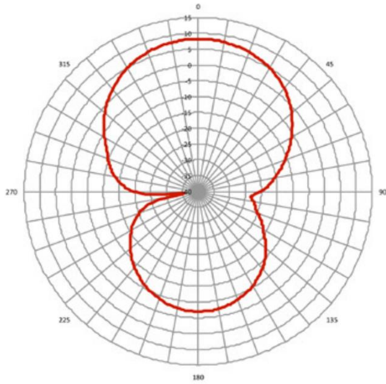
図 3: 860 MHz アンテナ放射パターン - 垂直面
