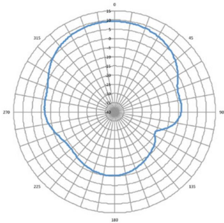
図 4: 902 MHz アンテナ放射パターン - 水平面
