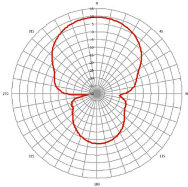
図 9: 928 MHz アンテナ放射パターン - 垂直面
