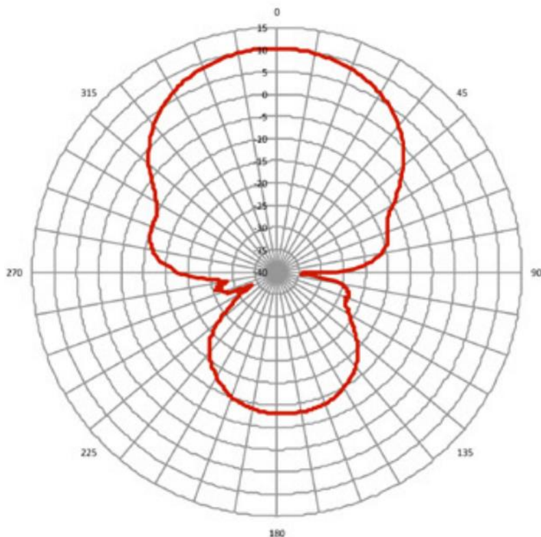
図 11: 960 MHz アンテナ放射パターン - 垂直面
