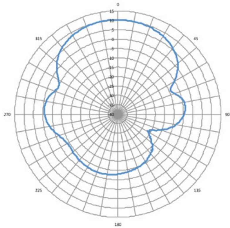
図 10 : 960 MHz アンテナ放射パターン - 水平面
