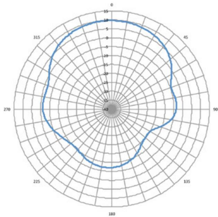
図 6: 910 MHz アンテナ放射パターン - 水平面
