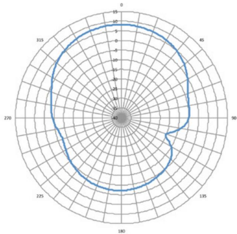
図 2: 860 MHz アンテナ放射パターン - 水平面
