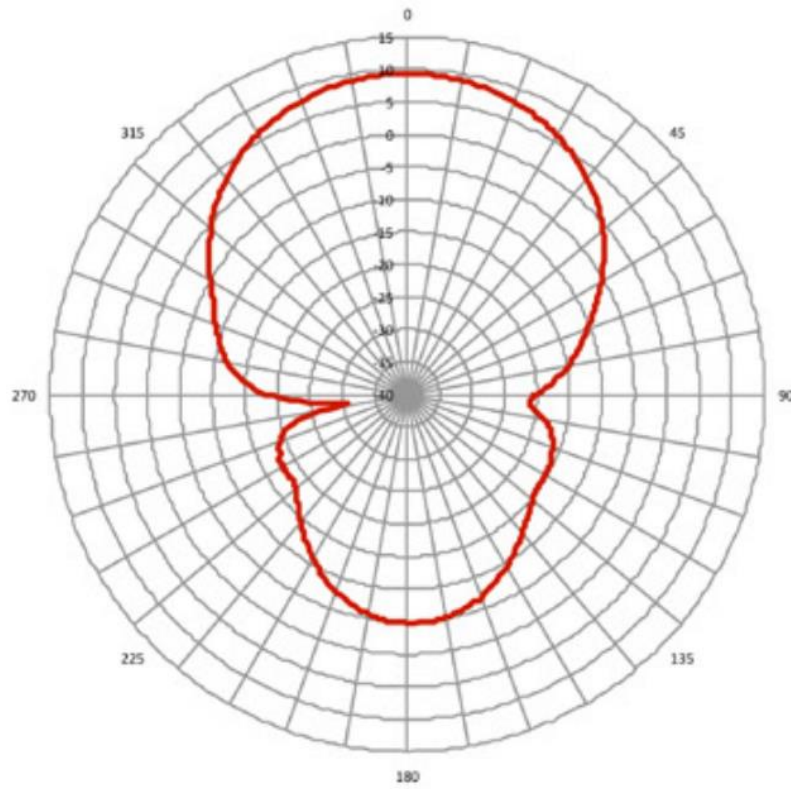
図 5: 902 MHz アンテナ放射パターン - 垂直面
