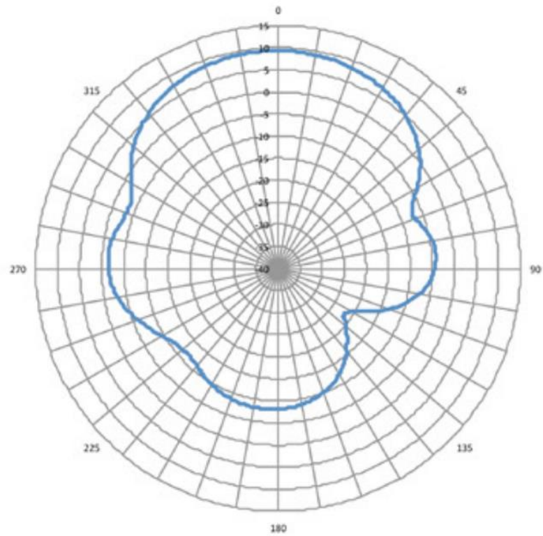
図 8: 928 MHz アンテナ放射パターン - 水平面
