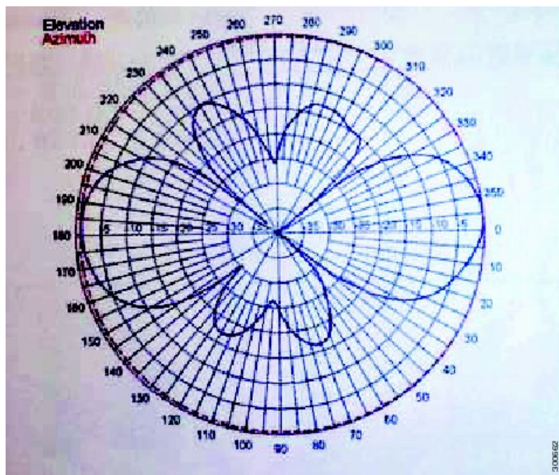
図 2: 屋外用無指向性アンテナの放射パターン
