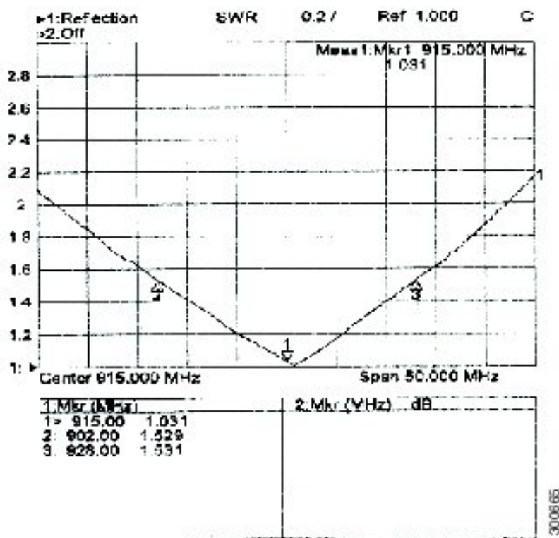
図 1: 屋外用無指向性アンテナの周波数パターン
