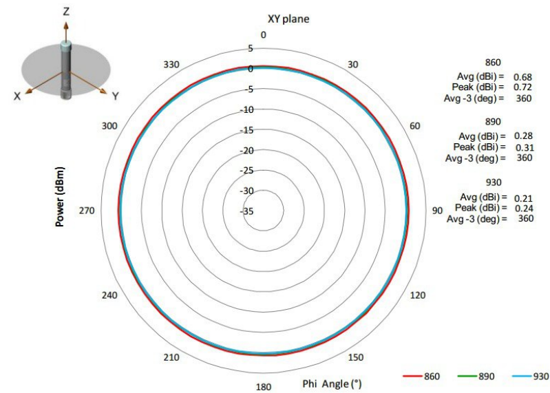
図 3: 放射パターン - 水平面
