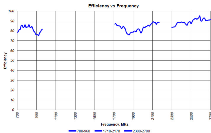
図 10: 効率
