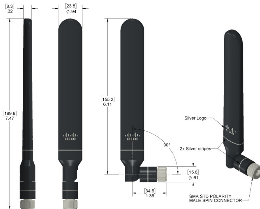
図 2: 機械図面
