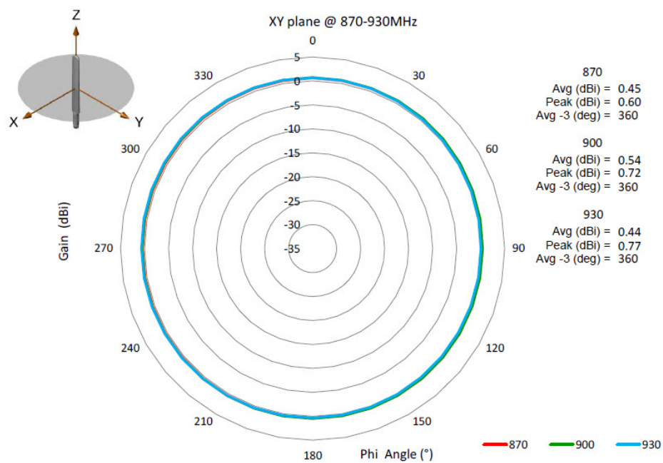
図 6: XY平面 @ 870 ~ 930 MHz
