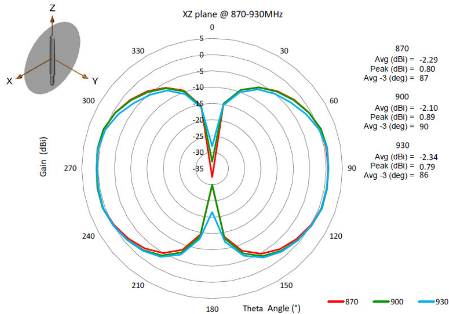
図 7: XZ 平面 @ 870 ~ 930 MHz
