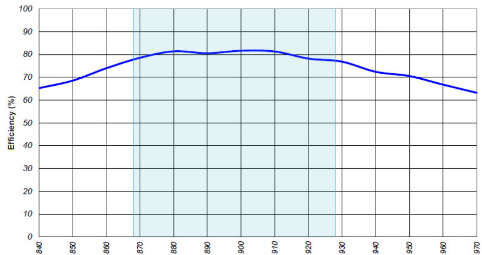
図 4: 効率と周波数
