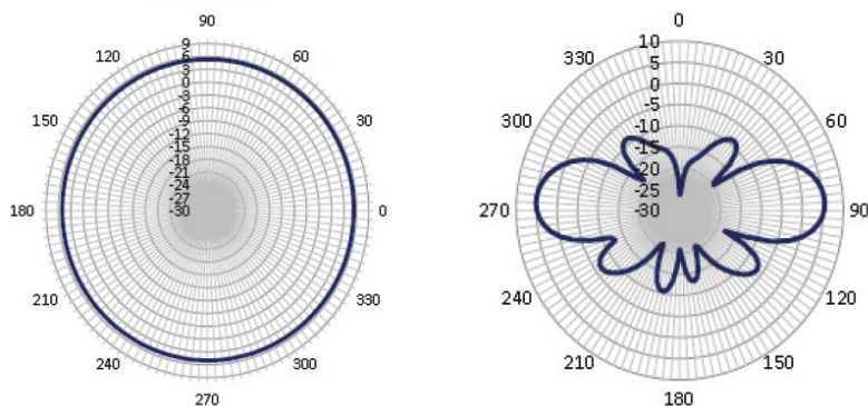
図 8: 928 MHz 放射パターン
