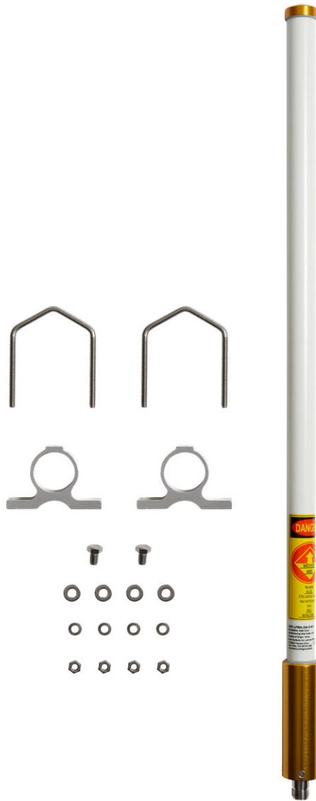
図 9: アンテナの取り付けコンポーネント
