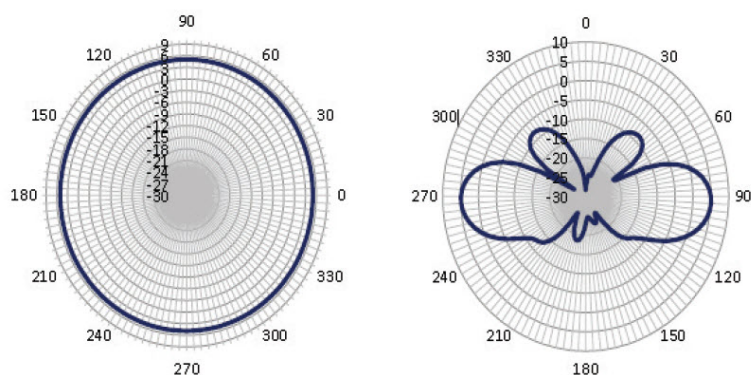
図 4: 869 MHz 放射パターン
