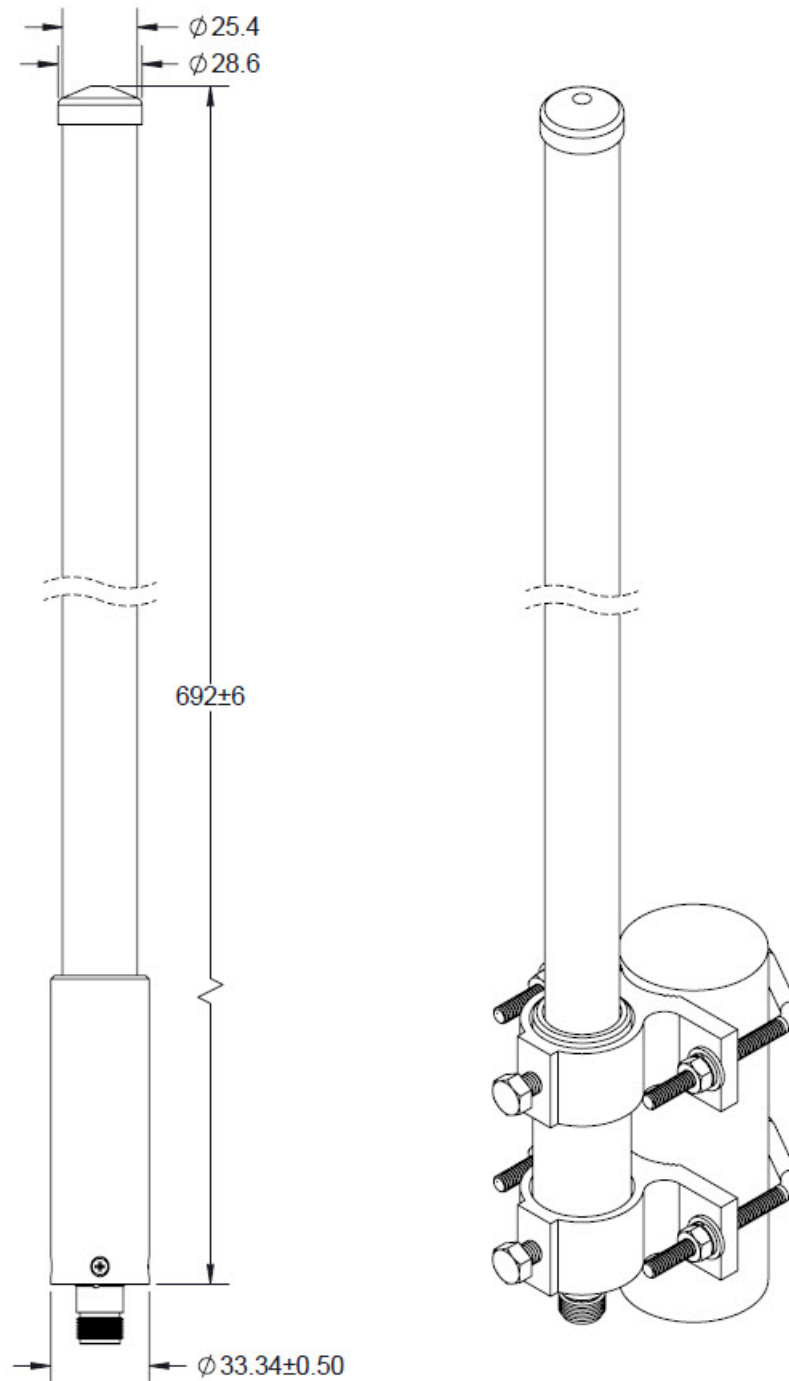
図 2: 寸法
