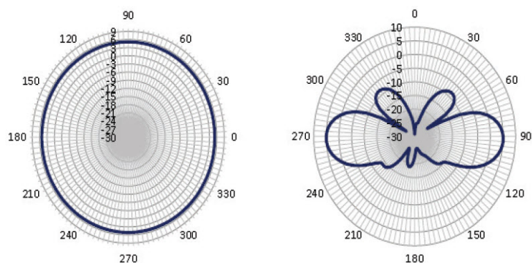
図 4: 869 MHz 放射パターン
