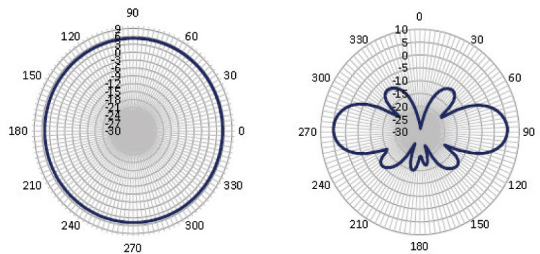
図 7: 914 MHz 放射パターン
