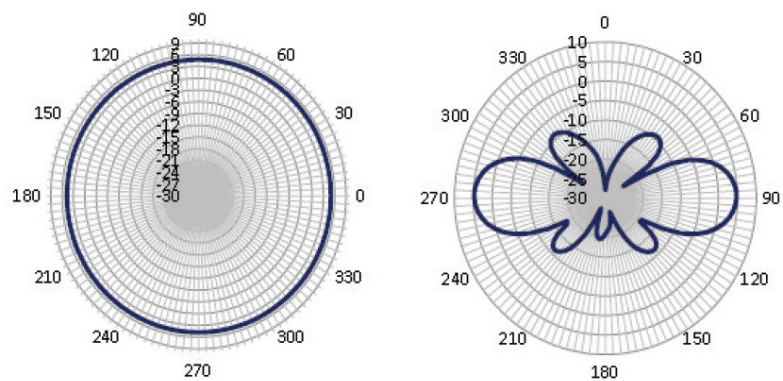
図 7: 914 MHz 放射パターン
