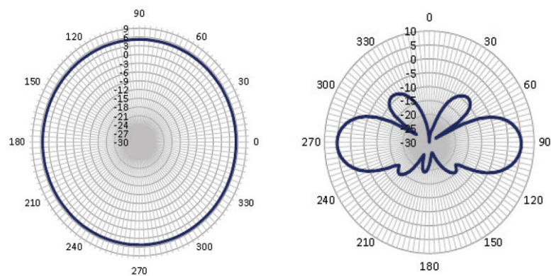
図 6: 902 MHz 放射パターン
