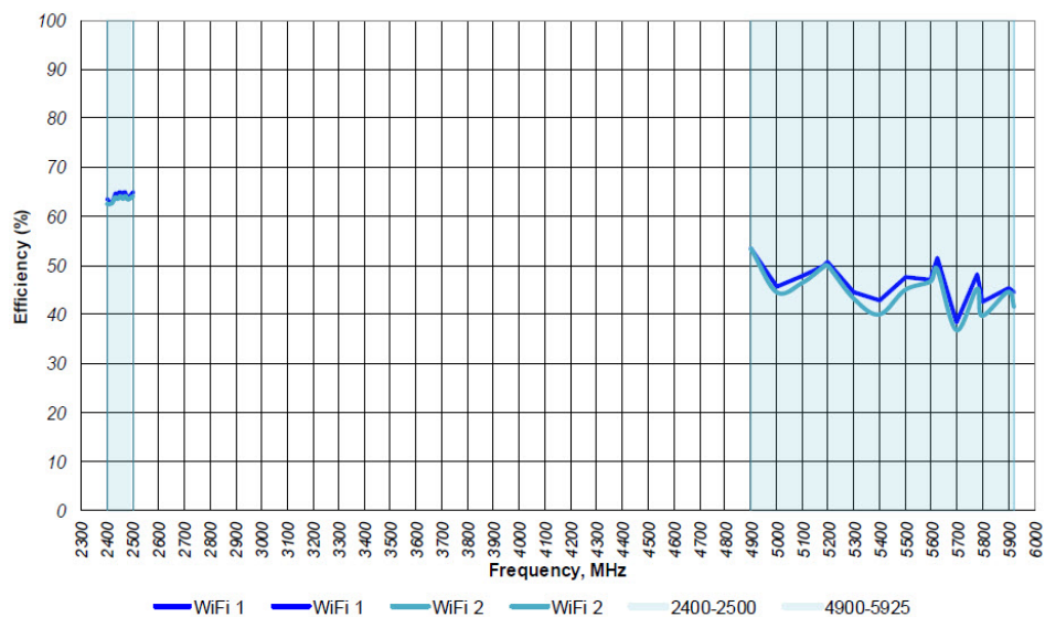
図 16: (Wi-Fi 1&amp;2) 2ft RG-316、Ø24in GP で測定
