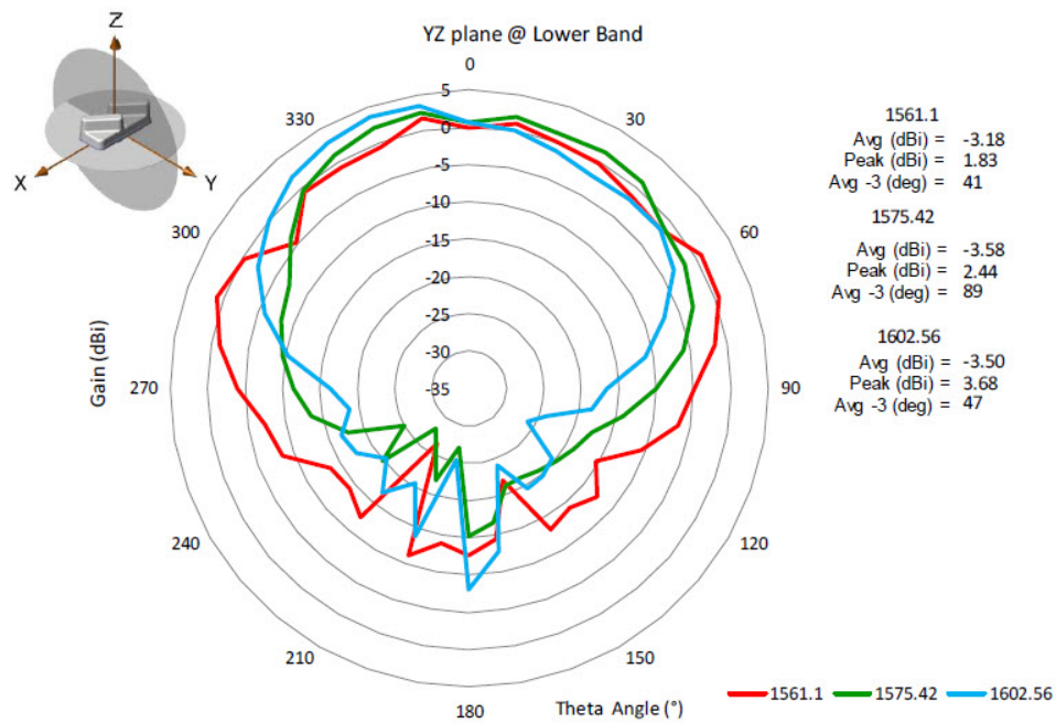
図 31 : YZ 平面 @ 低帯域
