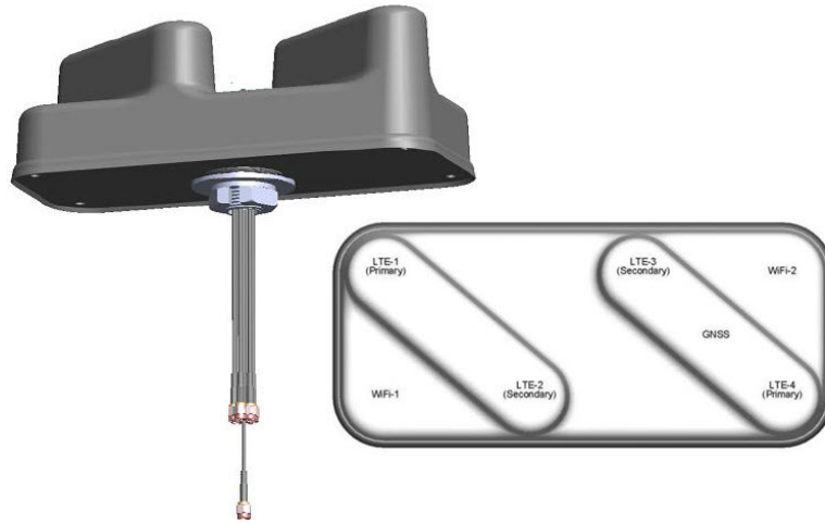
図 1: アンテナ写真
