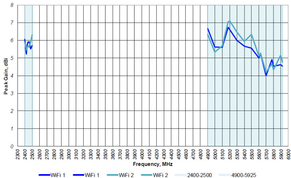
図 15: (Wi-Fi 1&amp;2) 2ft RG-316、Ø24in GP で測定
