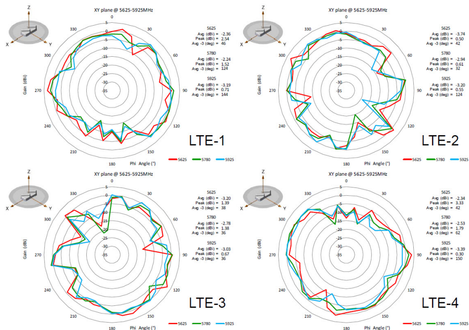
図 22: XY 平面 @ 5625 ~ 5925 MHz
