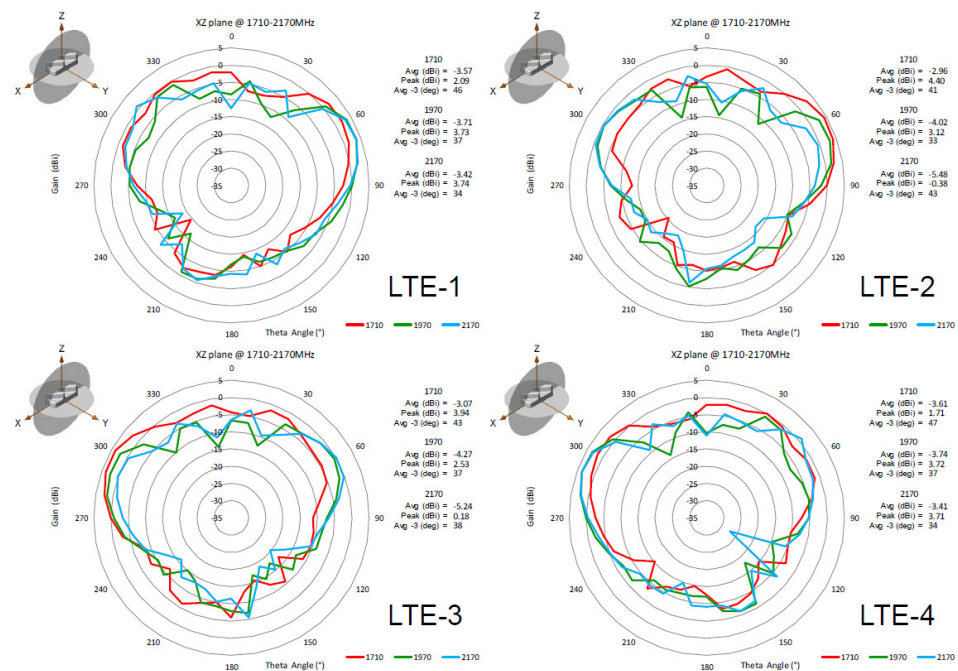
図 24: XZ 平面 @ 1710 ~ 2170 MHz
