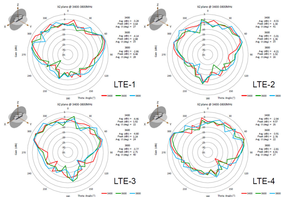
図 26: XZ 平面 @ 3400 ~ 3800 MHz
