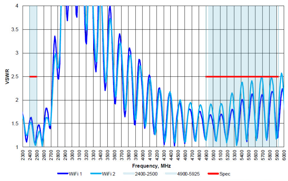
図 4: (Wi-Fi 1&2) 2ft RG-316、Ø24in GP で測定
