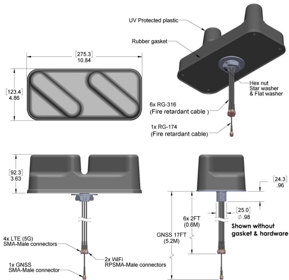
図 2: Cisco ANT-7-5G4WL2G1-O の機械的詳細
