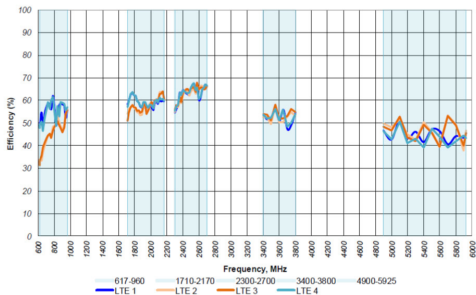
図 14: (LTE 1、2、3、4) 2ft RG-316、Ø24in GP で測定
