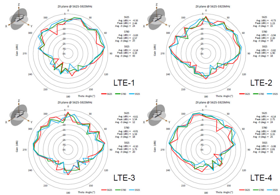
図 28: ZX 平面 @ 5625 ~ 5925 MHz
