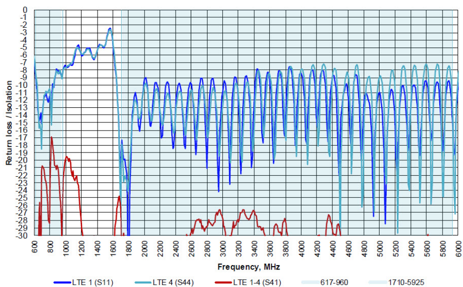
図 6: (LTE 1&4) 2ft RG-316、Ø24in GP で測定
