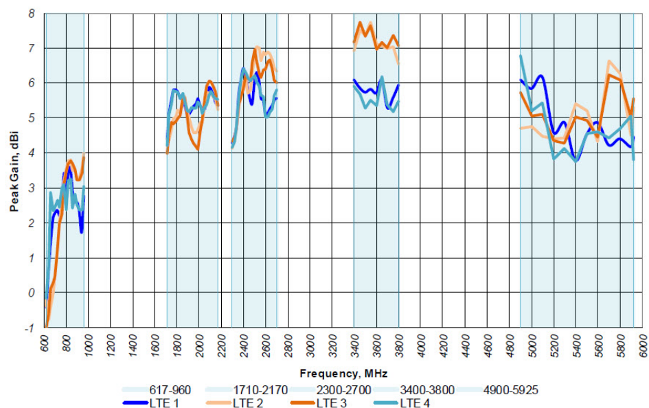
図 13: (LTE 1、2、3、4) 2ft RG-316、Ø24in GP で測定
