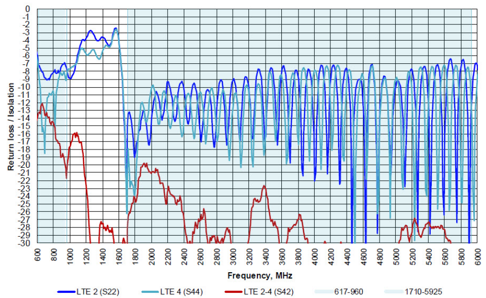
図 8: (LTE 2&amp;4) 2ft RG-316、Ø24in GP で測定
