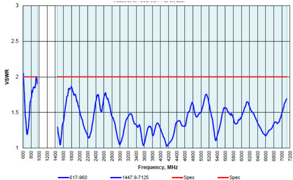
VSWR と周波数
