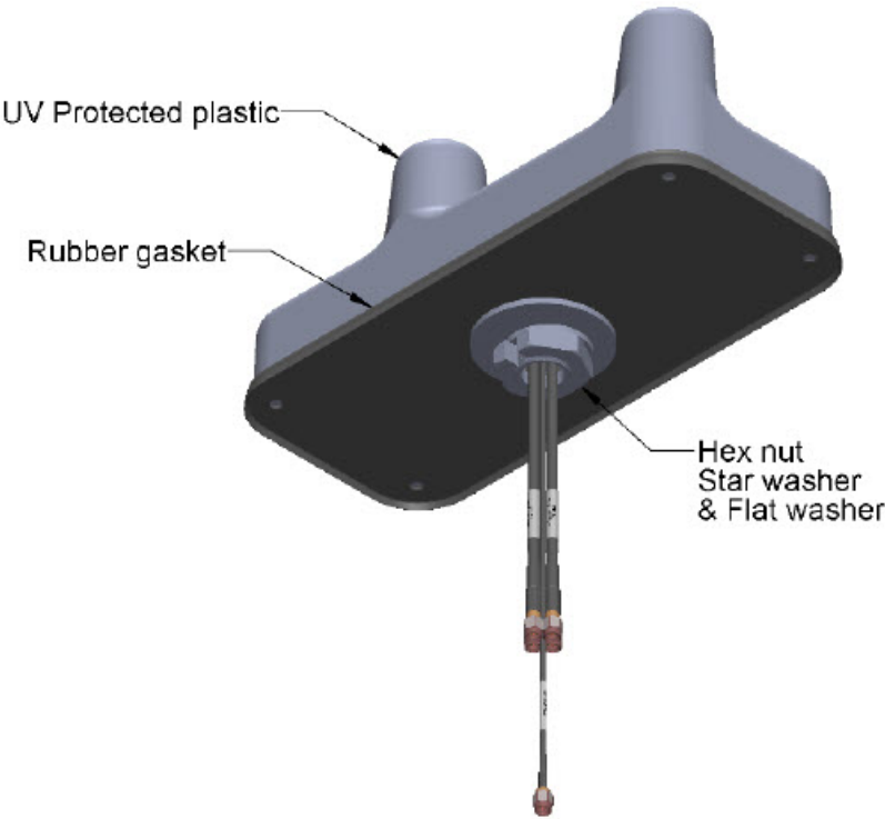
図 4: 機械の詳細 3
