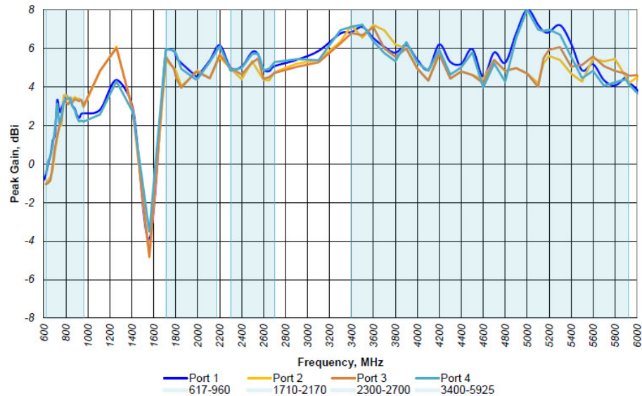
図 6: (LTE ポート 1 ~ 4) 2.3m (7.5フィート) LMR-195、Ø0.6M (2フィート) GP で測定
