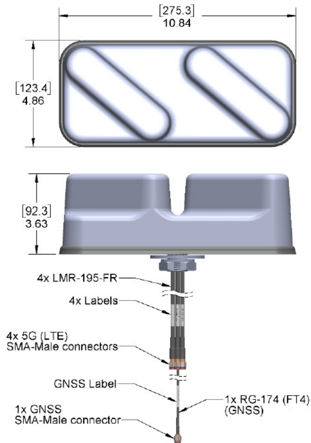
図 2: 機械の詳細 1
