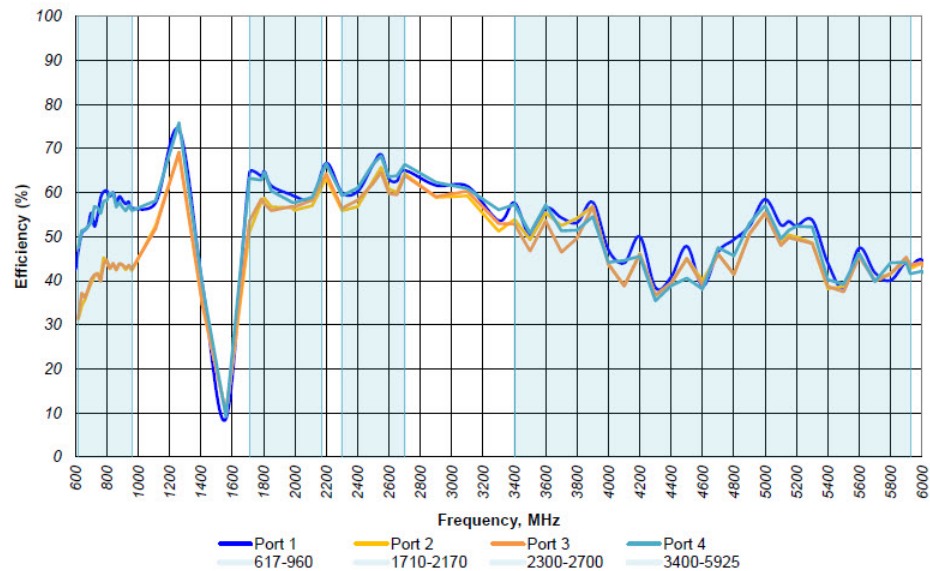
図 7: (LTE ポート 1 ~ 4) 2.3m (7.5フィート) LMR-195、Ø0.6M (2フィート) GP で測定
