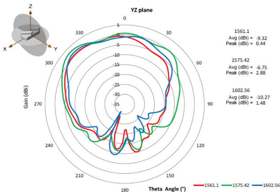
図 9: YZ 平面: 6 インチケーブルによるパッシブ測定
