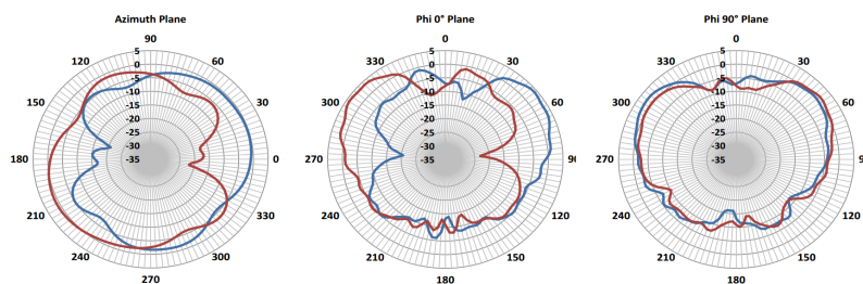
図 10: 2400 MHz WLAN アンテナ放射パターン
