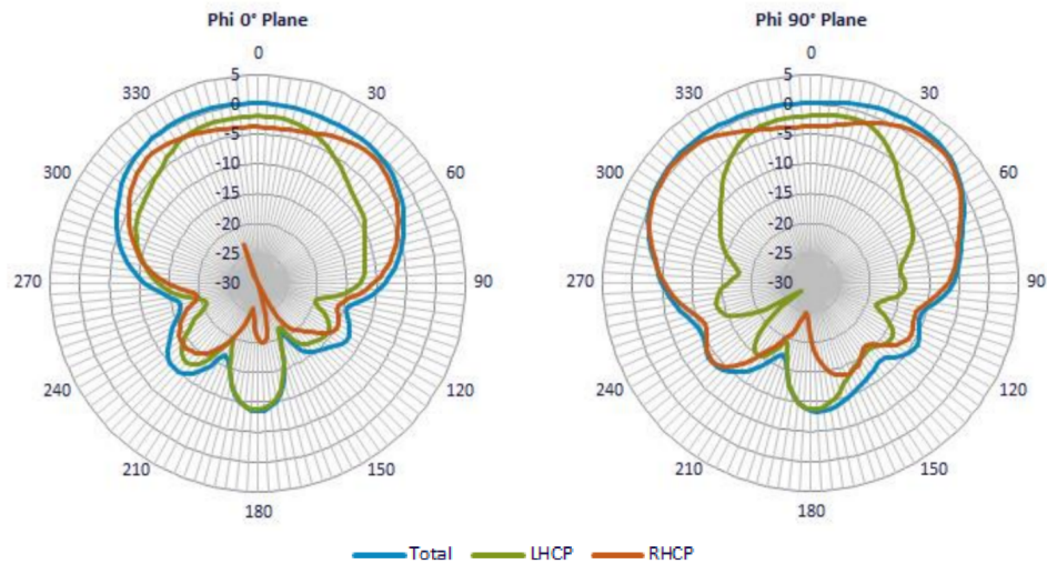
図 16: 1575 MHz GPS アンテナ放射パターン
