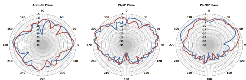
図 13 : 5150 MHz WLAN アンテナ放射パターン
