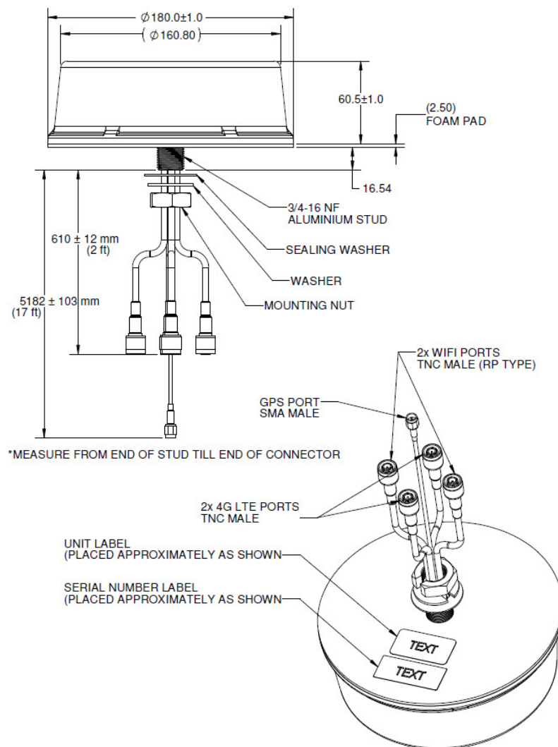
図 2: Cisco ANT-5-4G2WL2G1-0 の機械的詳細
