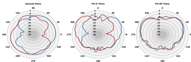
図 12 : 4900 MHz WLAN アンテナ放射パターン
