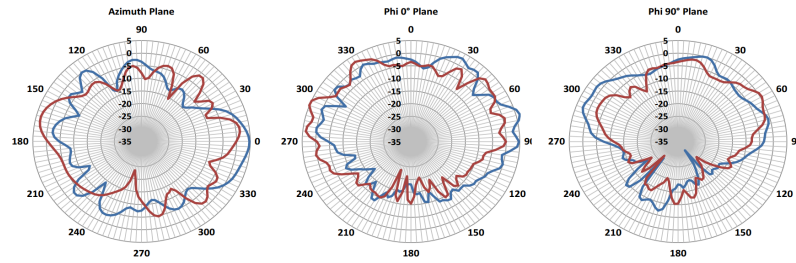
図 15: 5875 MHz WLAN アンテナ放射パターン
