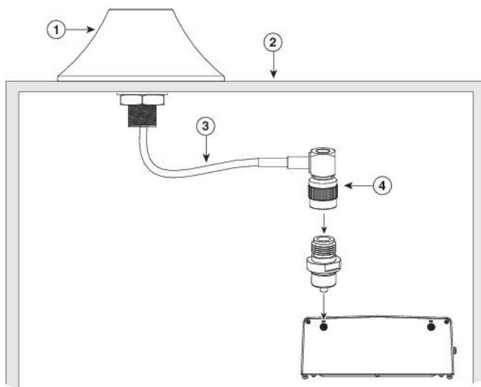
図 3: アンテナ詳細
