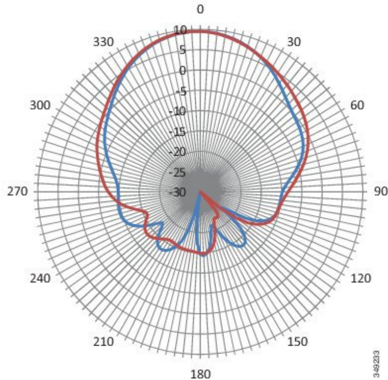
図 15: 2700 MHz アンテナ放射パターン - 垂直面
