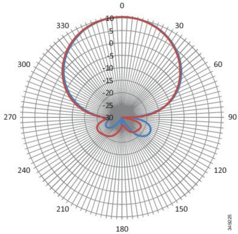
図 7: 960 MHz アンテナ放射パターン - 垂直面
