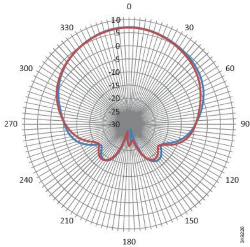
図 8: 1710 MHz アンテナ放射パターン - 水平面
