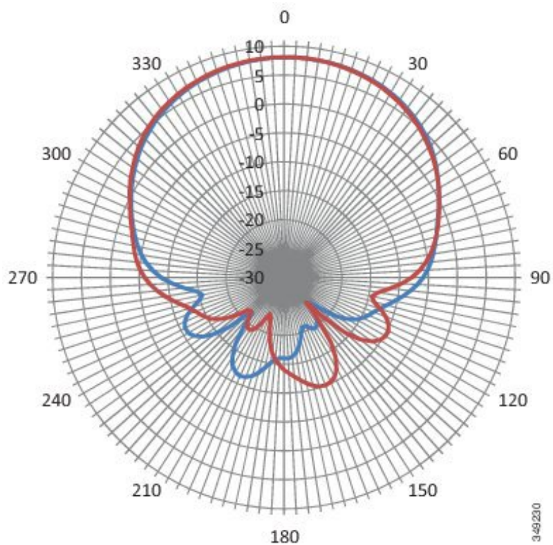
図 12: 2170 MHz アンテナ放射パターン - 水平面
