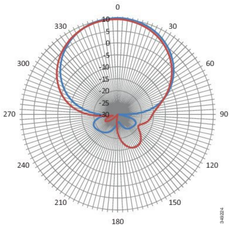
図 6 : 960 MHz アンテナ放射パターン - 水平面
