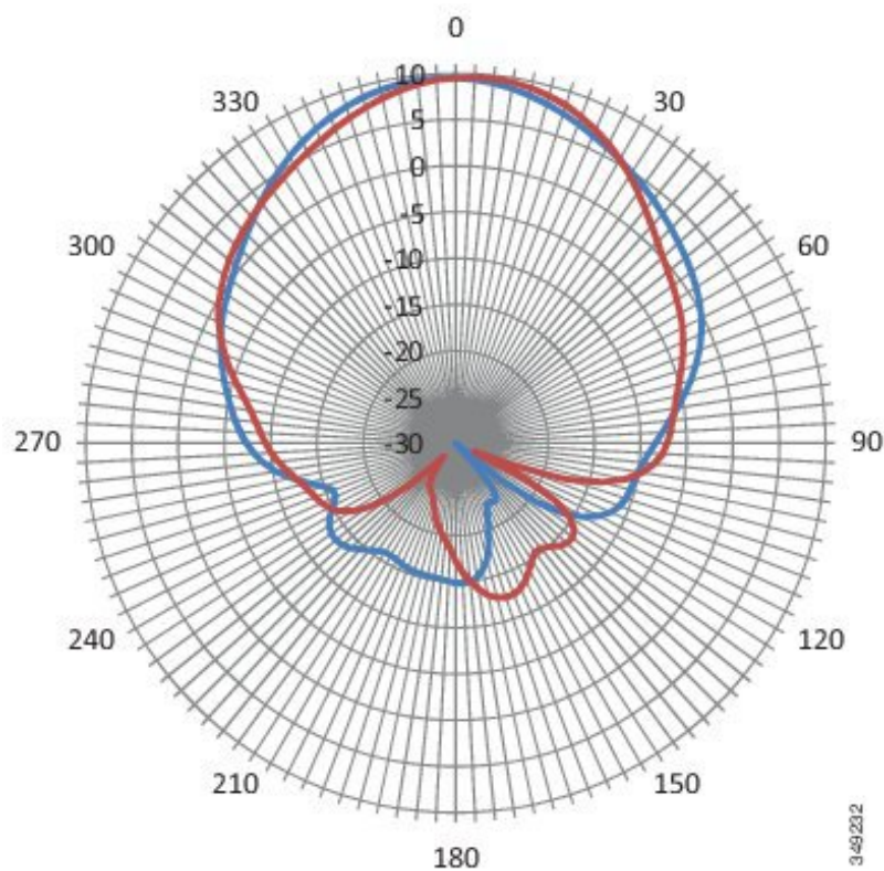
図 14 : 2700 MHz アンテナ放射パターン - 水平面
