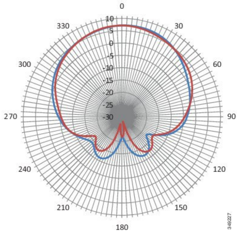
図 9: 1710 MHz アンテナ放射パターン - 垂直面
