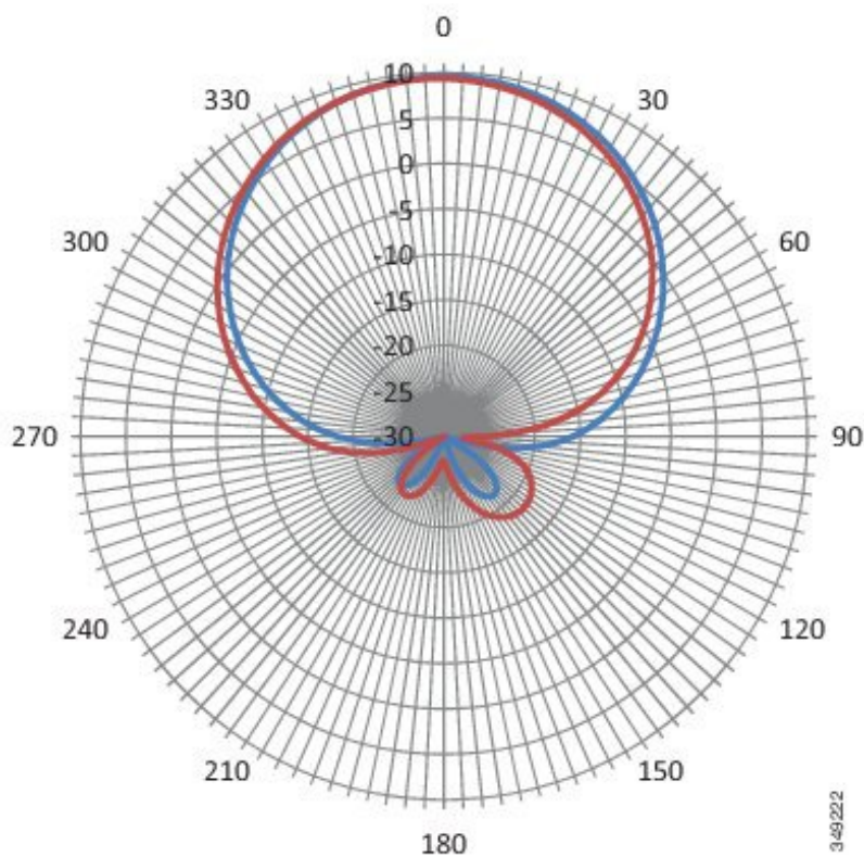
図 4: 880 MHz アンテナ放射パターン - 水平面
