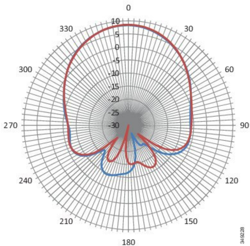
図 10: 1950 MHz アンテナ放射パターン - 水平面
