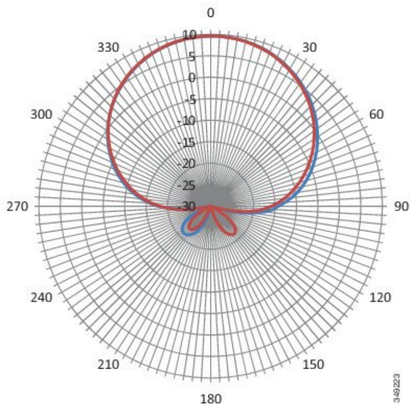
図 5: 880 MHz アンテナ放射パターン - 垂直面
