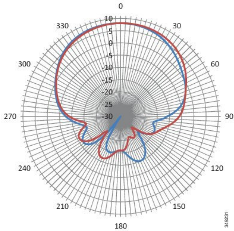
図 13: 2170 MHz アンテナ放射パターン - 垂直面
