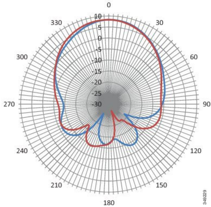
図 11 : 1950 MHz アンテナ放射パターン - 垂直面
