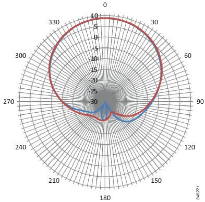
図 3: 698 MHz アンテナ放射パターン - 垂直面
