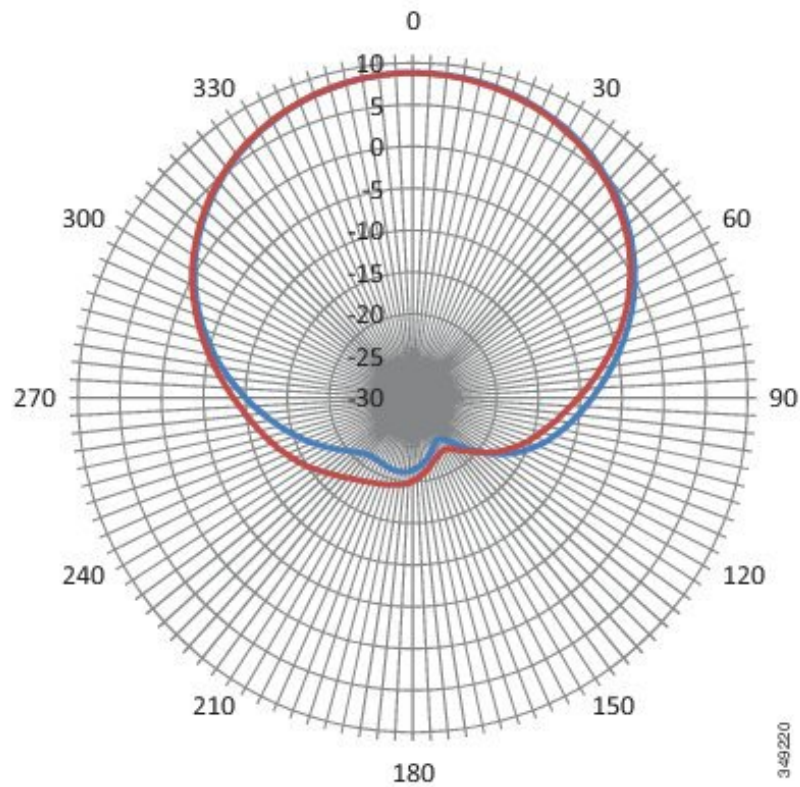
図 2: 698 MHz アンテナ放射パターン - 水平面
